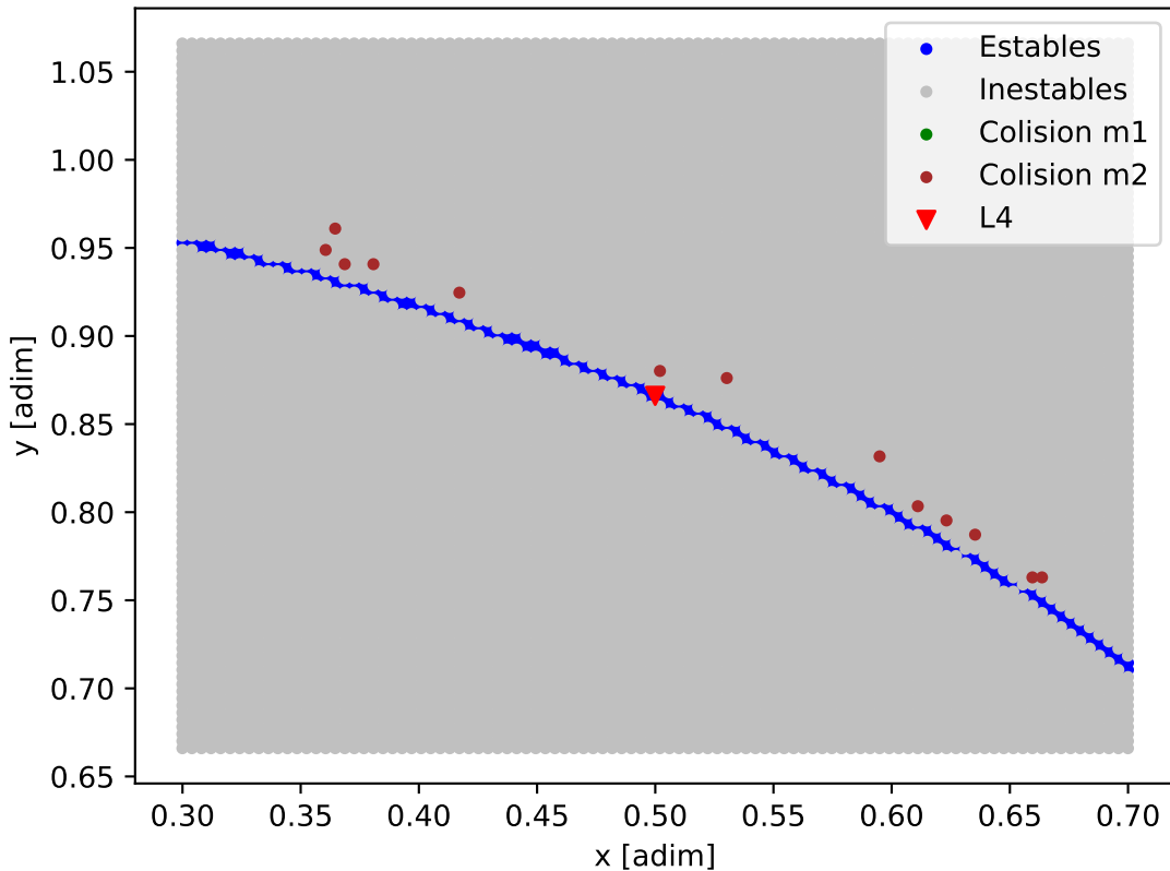
Mapa de estabilidad - TOI-406
