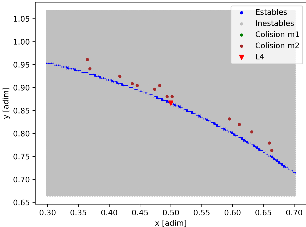
Mapa de estabilidad - Teegarden's_Star
