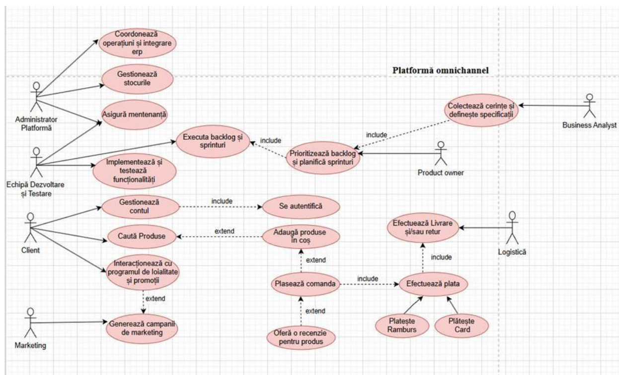
Figura 5. Diagrama cazurilor de utilizare – Platformă Omnichannel
