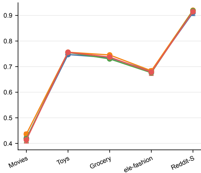
Macro-F1
