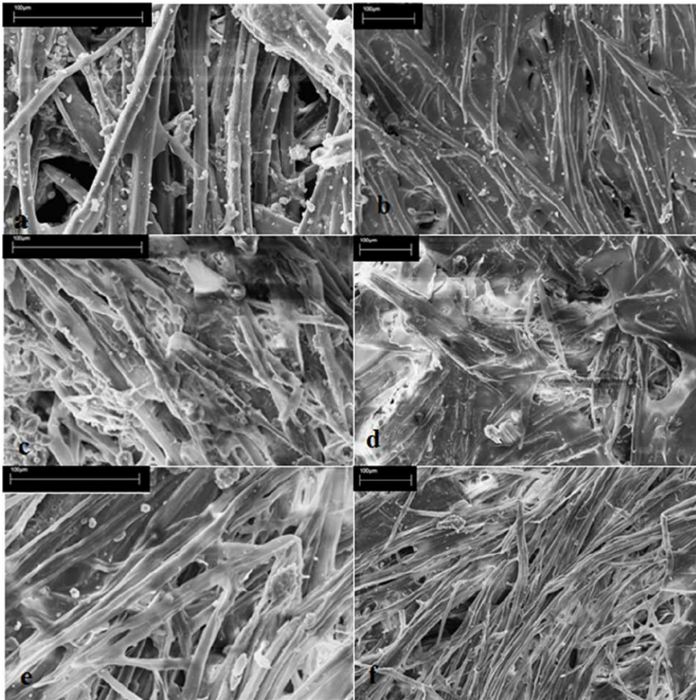
Figure 1.3: Immagini SEM delle fibre presenti nei nidi di Polistes dominula [1]
