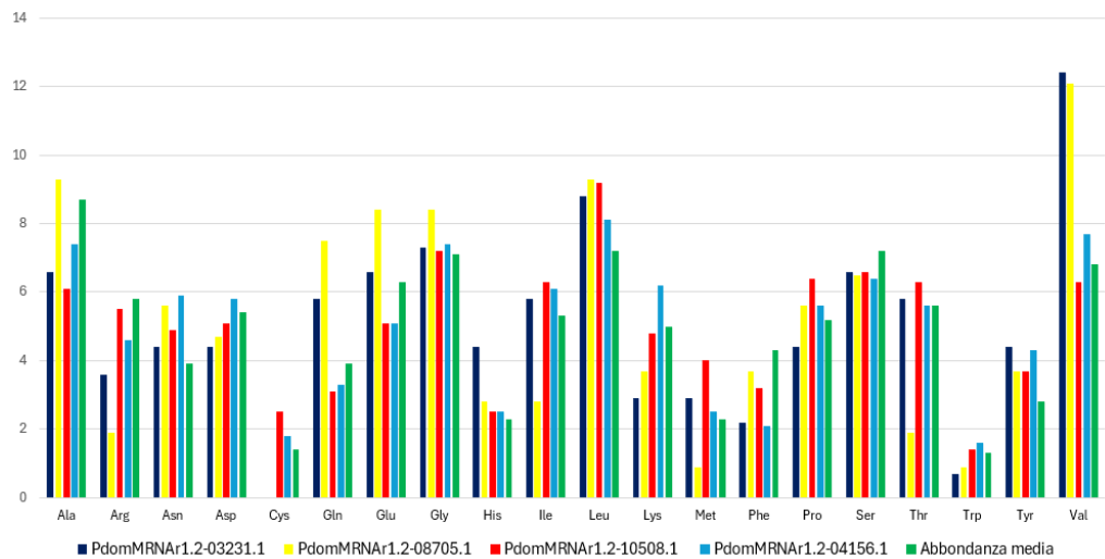
Figure 3.1: Abbondanze media degli amminoacidi messa a confronto con la abbondanza nelle quattro proteine di interesse
