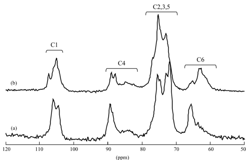
Figure 1.5: Spettri ^{13}\text{C} NMR di cellulosa in cui si evidenziano i diversi segnali dei carboni [3]
