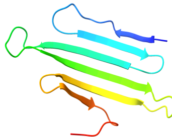
Figure 3.7: Struttura della proteina PdomMRNAr1.2-08705.1 eliminando la porzione ad alfa elica N-terminale
