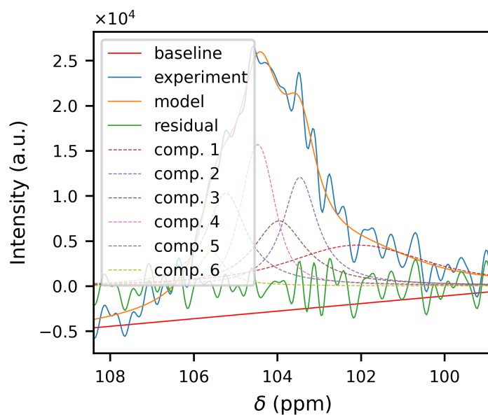
Figure 3.20: Fit della zona dei C1 per l'involucro di Vespa vulgaris (800 MHz)
