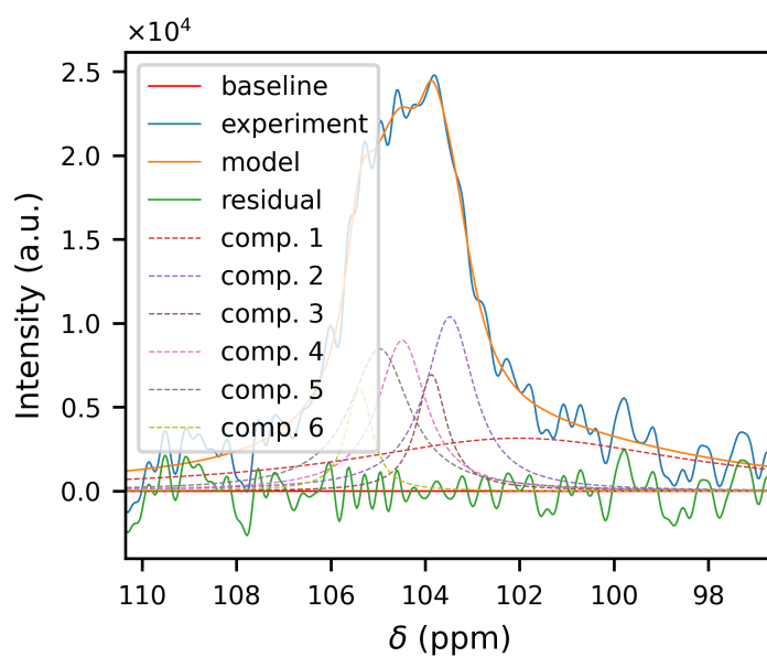
Figure 3.19: Fit della zona dei C1 per le celle di Vespa vulgaris (800 MHz)
