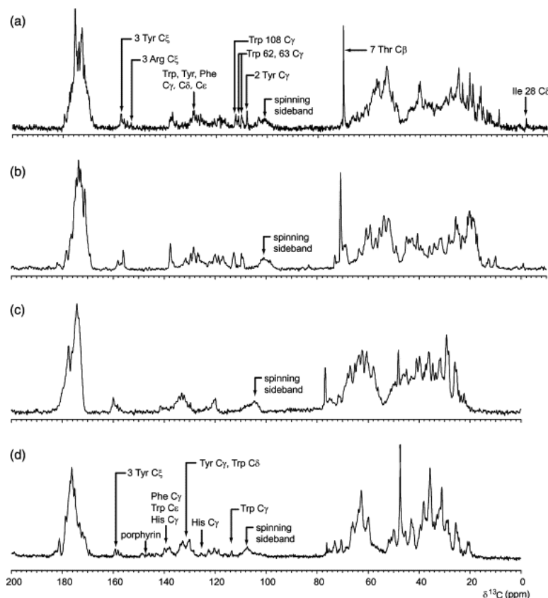
Figure 1.4: Spettri ^{13}\text{C} NMR di proteine nanocristalline: lisozima, streptavidina, ribonucleasi A e citocromo c (riprodotta da [2])
