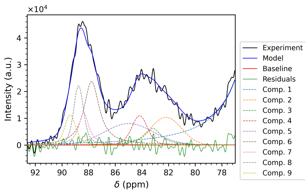
Figure 3.22: Fit della zona dei C 4 del campione più nuovo di Polistes dominula (800 MHz)
