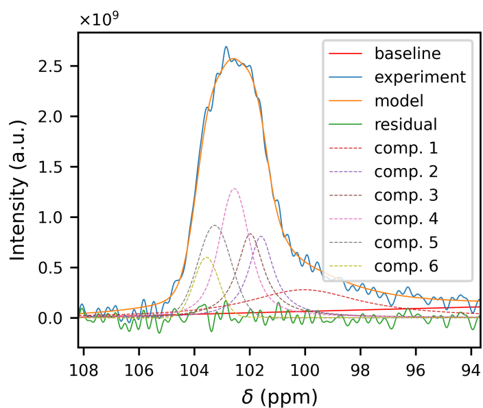
Figure 3.12: Fit della zona dei C1 per il campione più nuovo di Polistes dominula (700 MHz)
