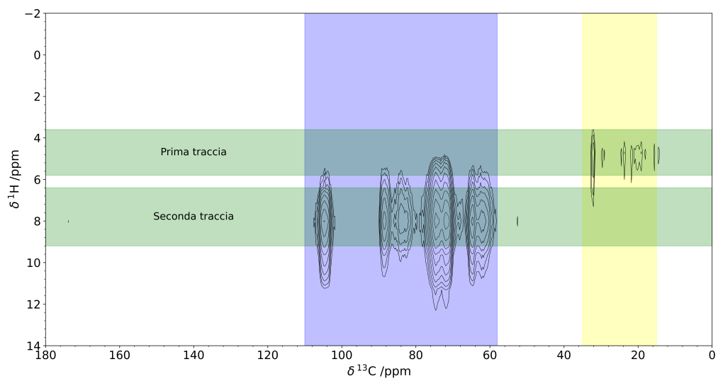
Figure 2.10: Spettro bidimensionale Polistes dominula
