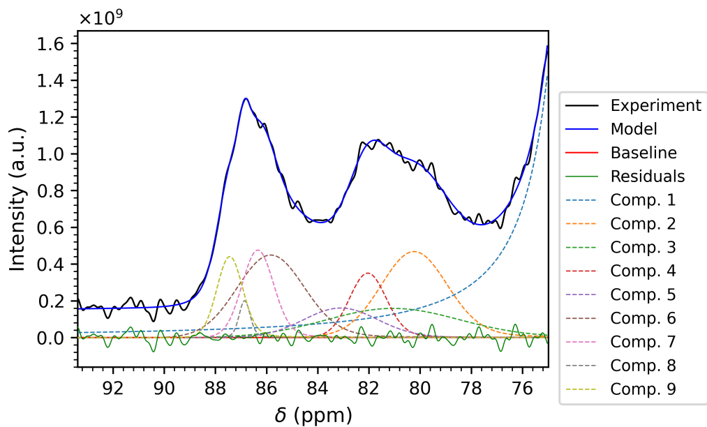
Figure 3.23: Fit della zona dei C4 del campione più vecchio di Polistes gallicus (700MHz)
