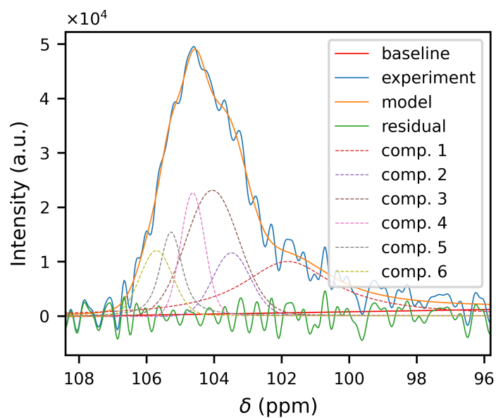
Figure 3.17: Fit della zona dei C1 per l'involucro di Vespa crabro (800 MHz)
