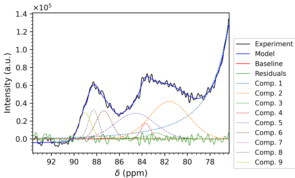
Figure 3.25: Fit della zona dei C 4 delle celle di Vespa Crabro (800 MHz)
