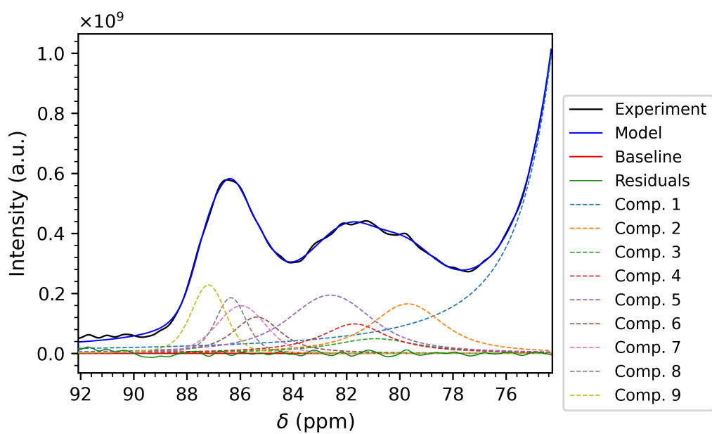
Figure 3.24: Fit della zona dei C4 del campione più nuovo di Polistes gallicus (700 MHz)
