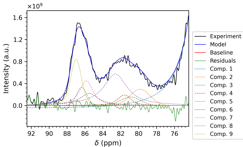
Figure 3.21: Fit della zona dei C 4 del campione più nuovo di Polistes dominula (700 MHz)
