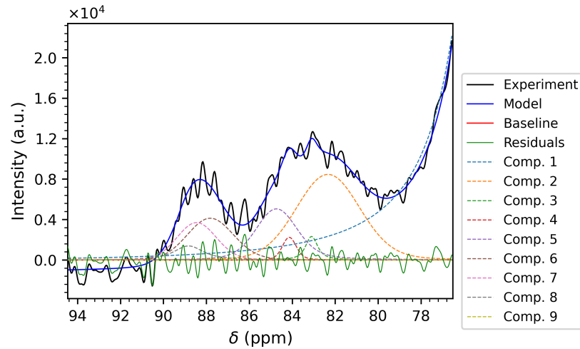
Figure 3.27: Fit della zona dei C 4 delle celle di Vespula vulgaris (800 MHz)
