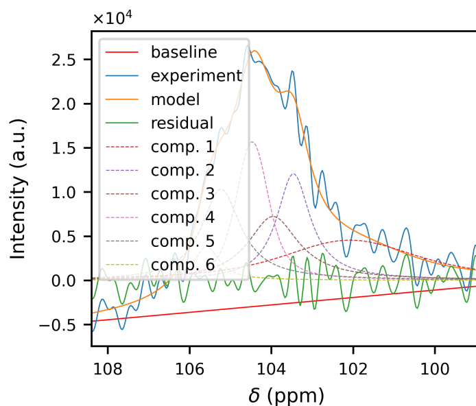
Figure 3.19: Fit della zona dei C1 per l'involucro di Vespula vulgaris (800 MHz)
