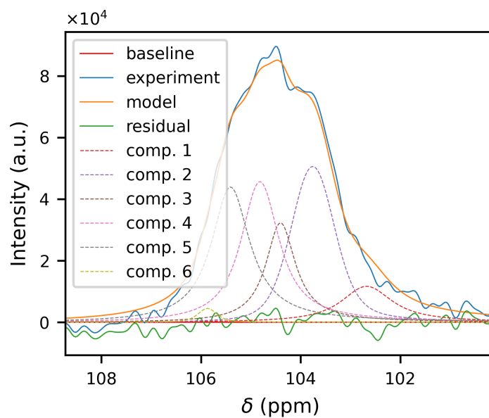
Figure 3.13: Fit della zona dei C1 per il campione più nuovo di Polistes dominula (800 MHz)
