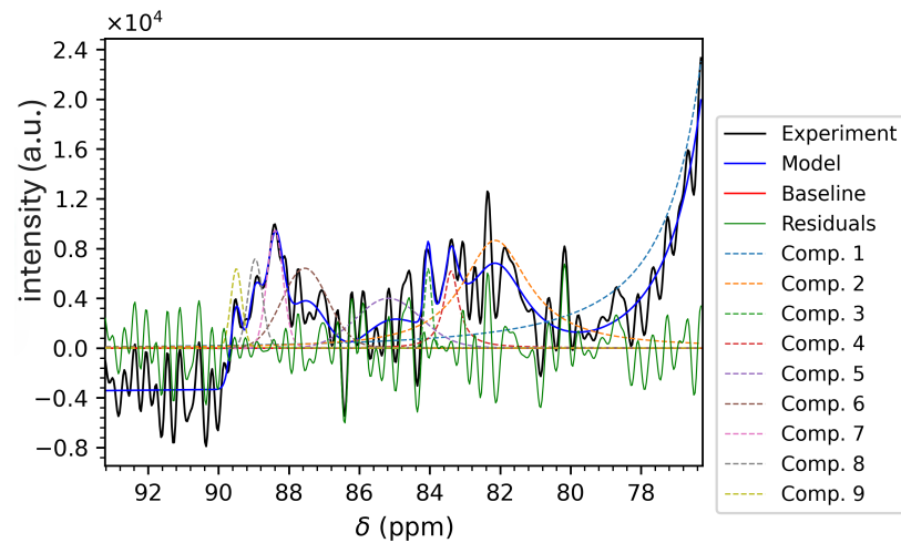
Figure 3.28: Fit della zona dei C 4 dell'involucro di Vespula vulgaris (800 MHz)
