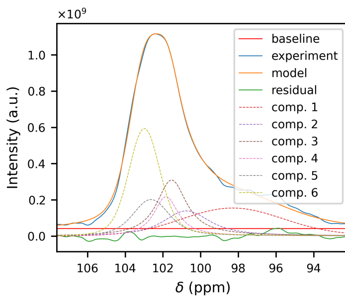
Figure 3.15: Fit della zona dei C1 per il campione più nuovo di Polistes gallicus (700 MHz)
