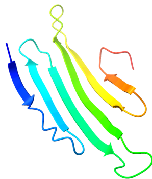
Figure 3.5: Struttura della proteina PdomMRNAr1.2-03231.1 eliminando la porzione ad alfa elica
