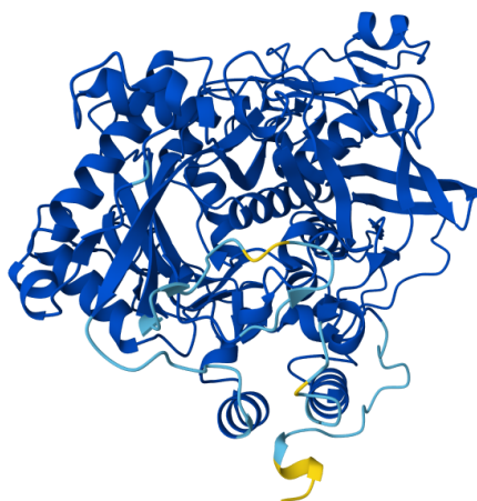
Figure 3.4: Struttura della proteina PdomMRNAr1.2-04156.1 predetta con Alphafold
