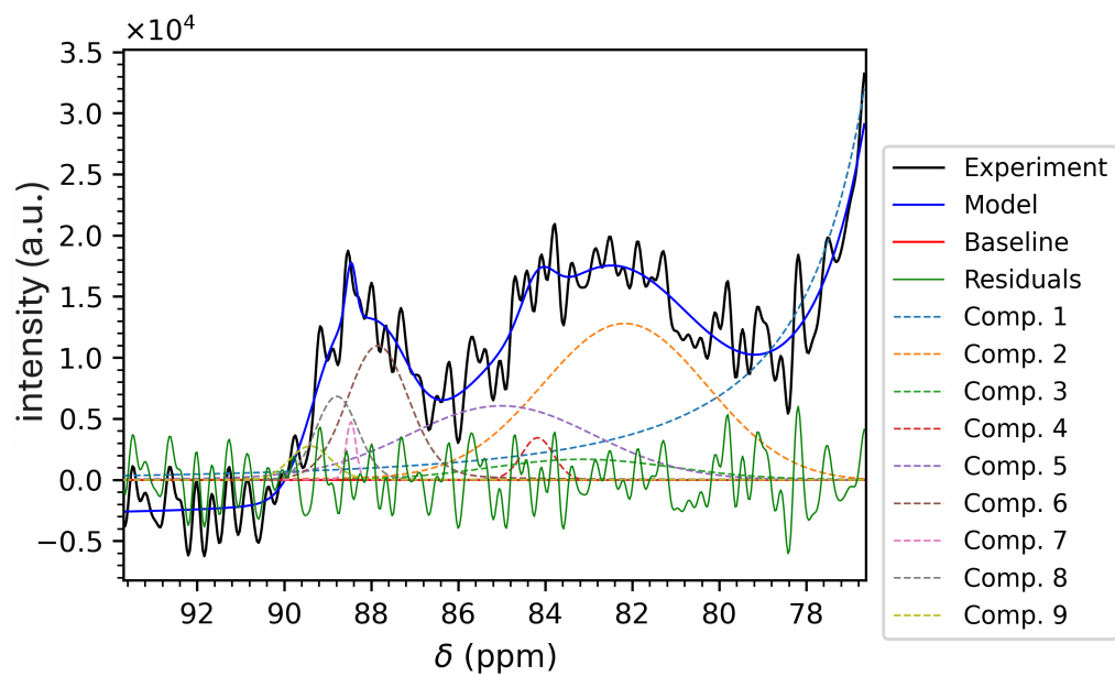
Figure 3.26: Fit della zona dei C 4 dell'involucro di Vespa crabro (800 MHz)
