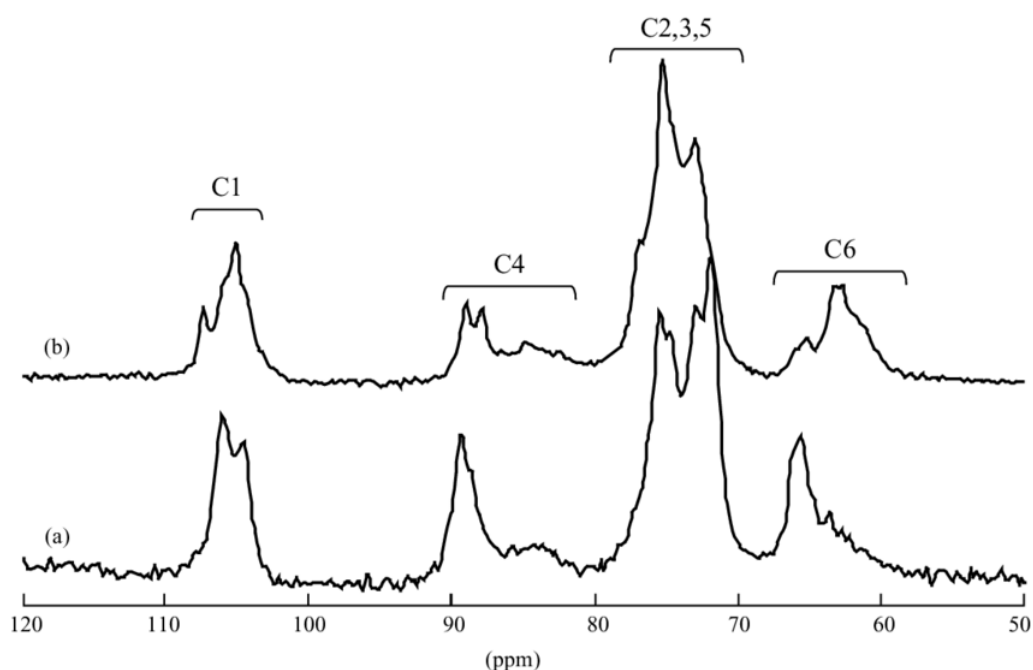
Figure 1.4: Spettri ^{13}\text{C} NMR di cellulosa in cui si evidenziano i diversi segnali dei carboni [3]
