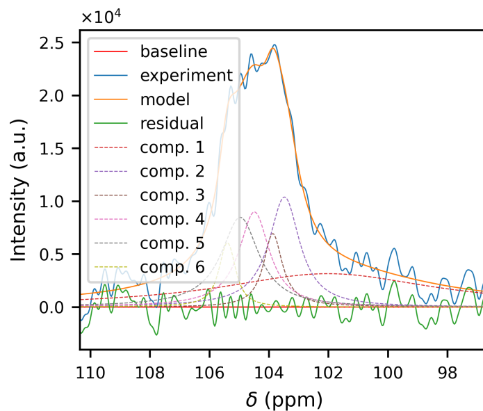
Figure 3.18: Fit della zona dei C1 per le celle di Vespula vulgaris (800 MHz)
