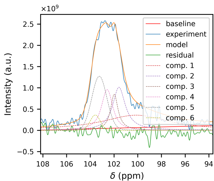
Figure 3.11: Fit della zona dei C1 per il campione più vecchio di Polistes dominula (700 MHz)
