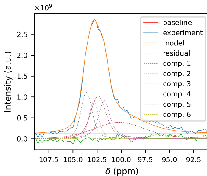
Figure 3.14: Fit della zona dei C1 per il campione più vecchio di Polistes gallicus (800 MHz)
