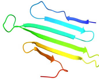
Figure 3.6: Struttura della proteina PdomMRNAr1.2-08705.1 eliminando la porzione ad alfa elica
