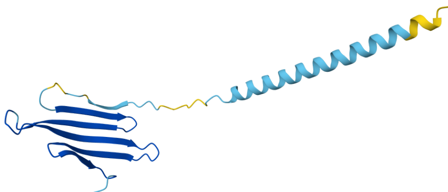
Figure 3.1: Struttura della proteina PdomMRNAr1.2-03231.1 predetta con Alphafold
