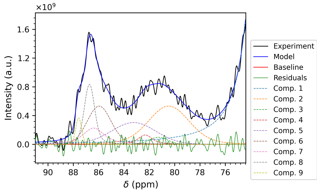
Figure 3.20: Fit della zona dei C4 del campione più vecchio di Polistes dominula (700 MHz)
