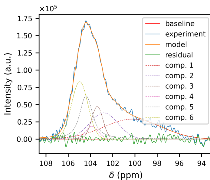
Figure 3.16: Fit della zona dei C1 per le celle di Vespa crabro (800 MHz)
