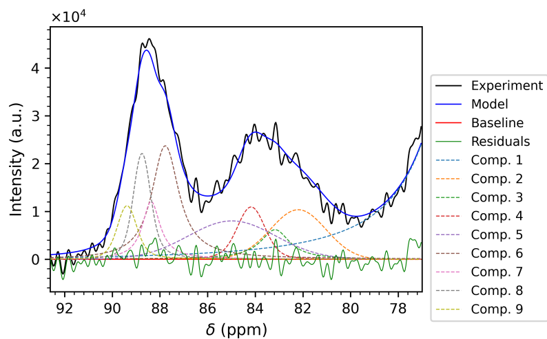
Figure 3.22: Fit della zona dei C 4 del campione più nuovo di Polistes dominula (800 MHz)
