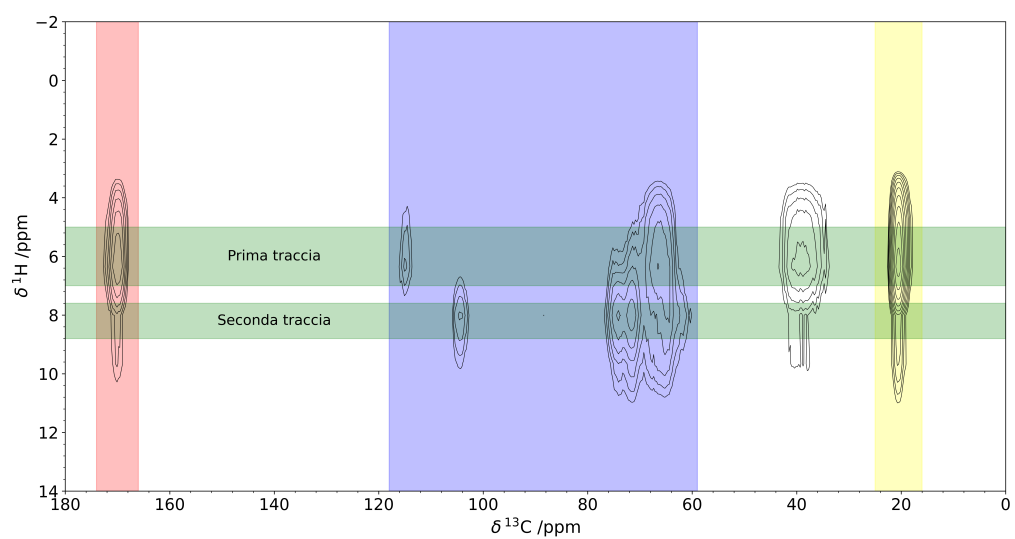
Figure 2.16: Spettro bidimensionale Vespula vulgaris
