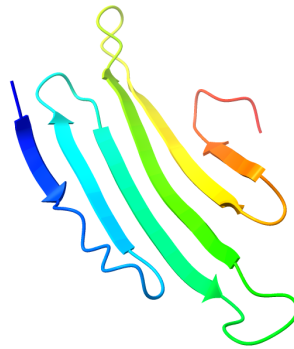
Figure 3.5: Struttura della proteina PdomMRNAr1.2-03231.1 eliminando la porzione ad alfa elica N-terminale
