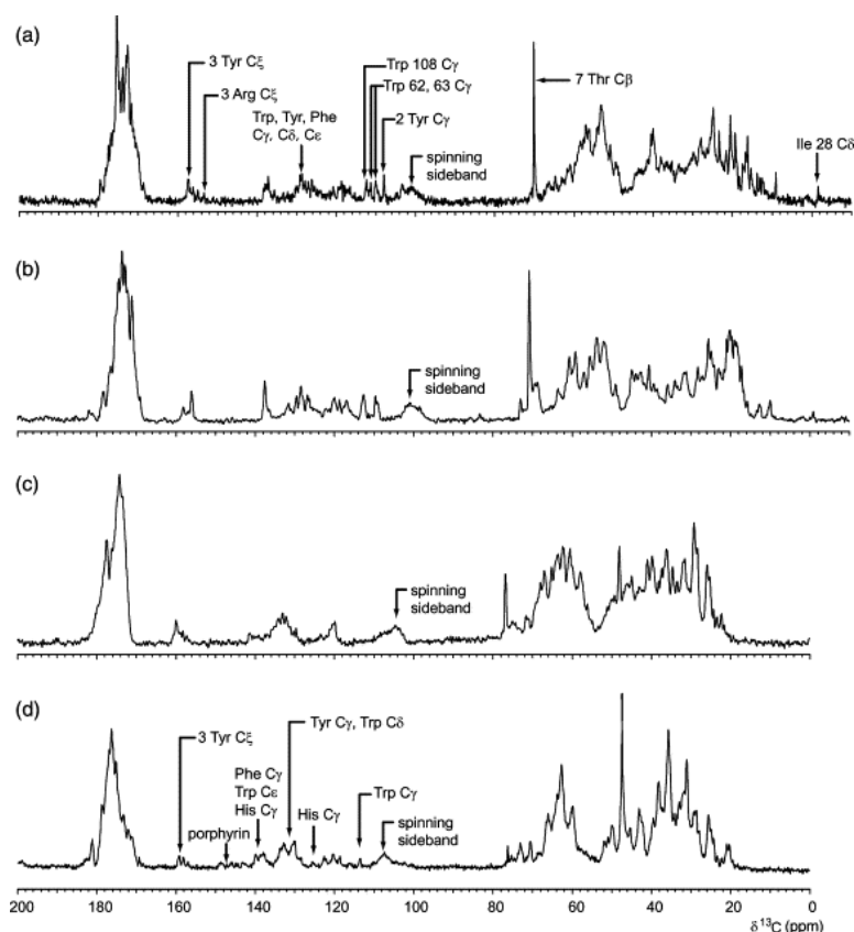
Figure 1.3: Spettri ^{13}\text{C} NMR di proteine nanocristalline: lisozima, streptavidina, ribonucleasi A e citocromo c (riprodotta da [2])
