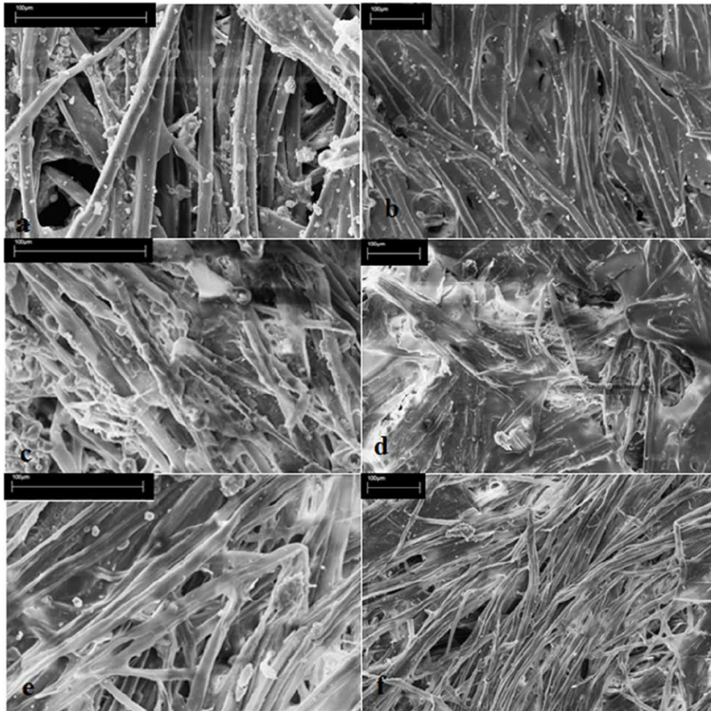
Figure 1.2: Immagini SEM delle fibre presenti nei nidi di Polistes dominula [2]
