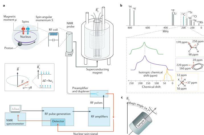
Figure 2.1: Schematica rappresentazione del funzionamento dello strumento
