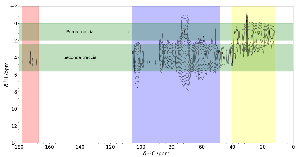
Figure 2.14: Spettro bidimensionale Polistes gallicus
