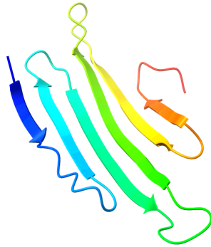
Figure 3.1: Struttura della proteina PdomMRNAr1.2-03231.1 eliminando la porzione ad alfa elica
