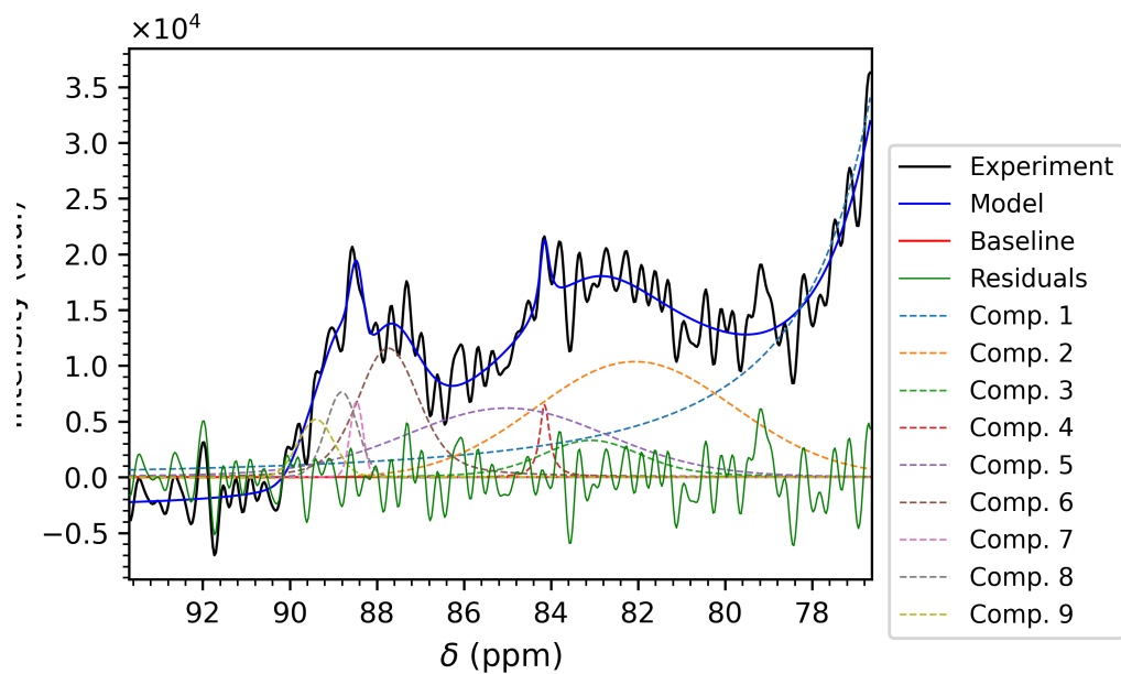
Figure 3.22: Fit della zona dei C 4 dell'involucro di Vespa crabro (800 MHz)
