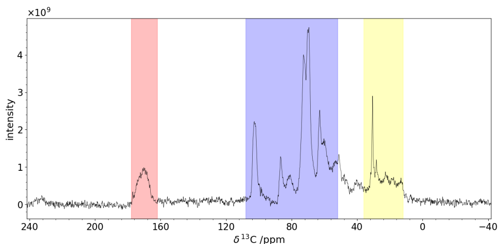
Figure 2.2: Spettro ^{13}\text{C} CP/MAS NMR del campione più vecchio di Polistes dominula (700MHz)
