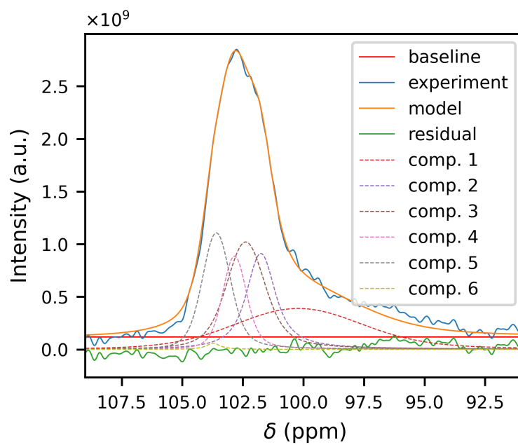
Figure 3.10: Fit della zona dei C_1 per il campione più vecchio di Polistes gallicus (800 MHz)
