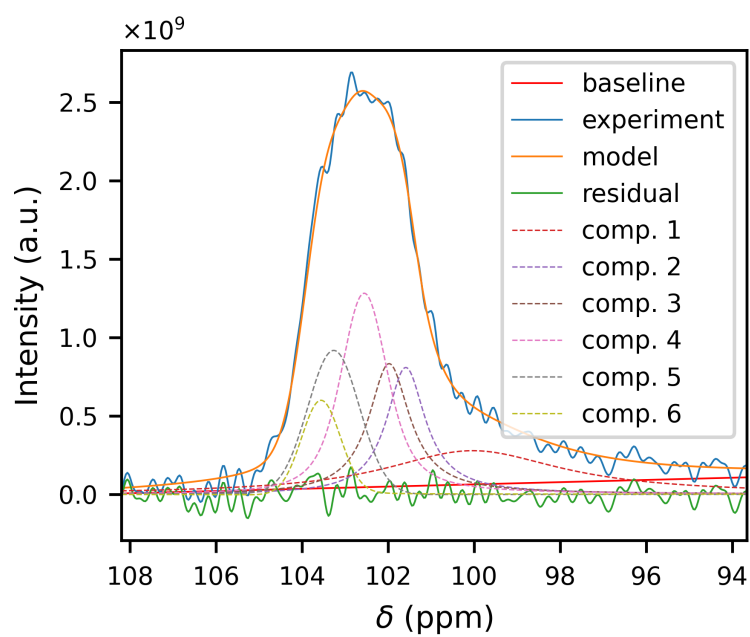
Figure 3.8: Fit della zona dei C1 per il campione più nuovo di Polistes dominula (700 MHz)
