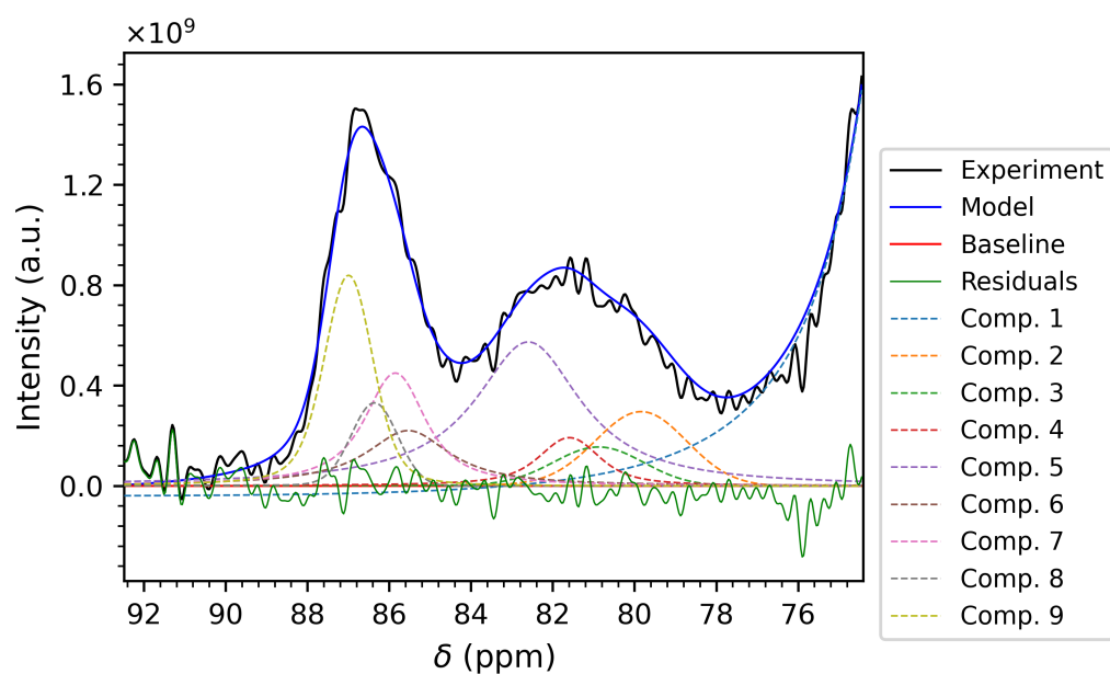
Figure 3.17: Fit della zona dei C 4 del campione più nuovo di Polistes dominula (700 MHz)
