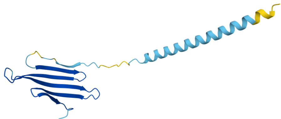
Figure 1.2: Struttura della proteina PdomMRNAr1.2-03231.1 predetta con Alphafold
