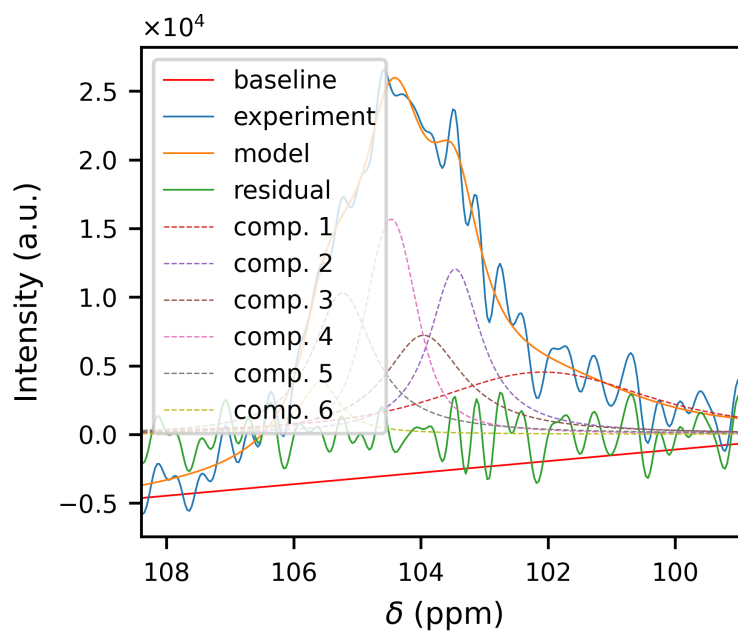
Figure 3.15: Fit della zona dei C1 per l'involucro di Vespa vulgaris (800 MHz)
