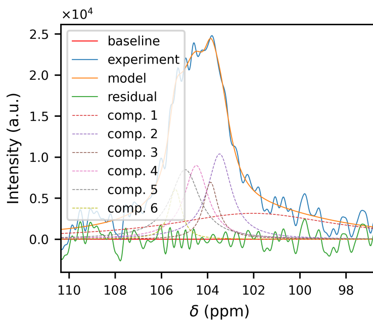
Figure 3.14: Fit della zona dei C1 per le celle di Vespa vulgaris (800 MHz)
