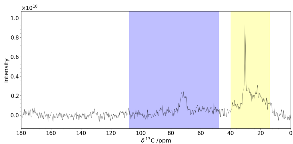
Figure 2.15: Prima traccia del segnale del protone Polistes gallicus
