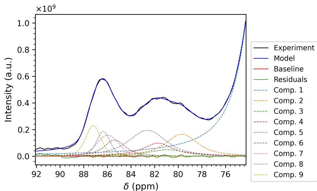
Figure 3.20: Fit della zona dei C 4 del campione più nuovo di Polistes gallicus (700 MHz)
