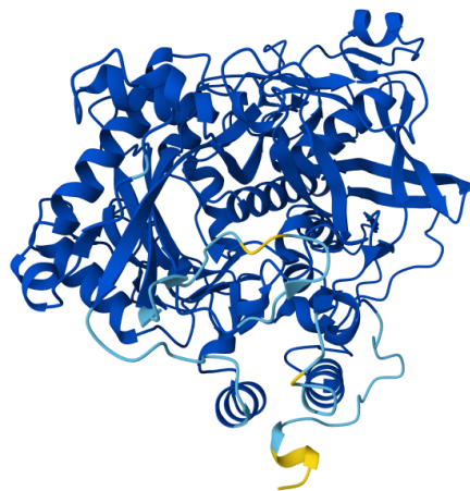
Figure 1.5: Struttura della proteina PdomMRNAr1.2-04156.1 predetta con Alphafold
