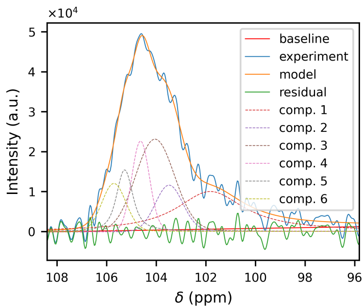
Figure 3.13: Fit della zona dei C1 per l'involucro di Vespa crabro (800 MHz)
