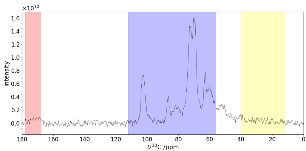
Figure 2.16: Seconda traccia del segnale del protone Polistes gallicus
