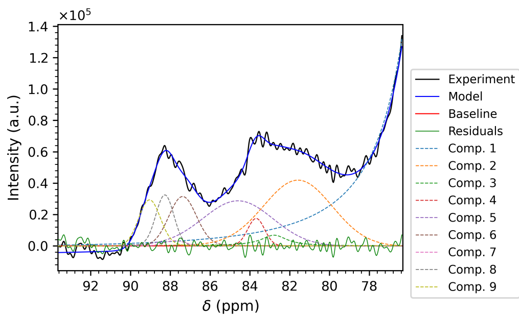
Figure 3.21: Fit della zona dei C 4 delle celle di Vespa Crabro (800 MHz)
