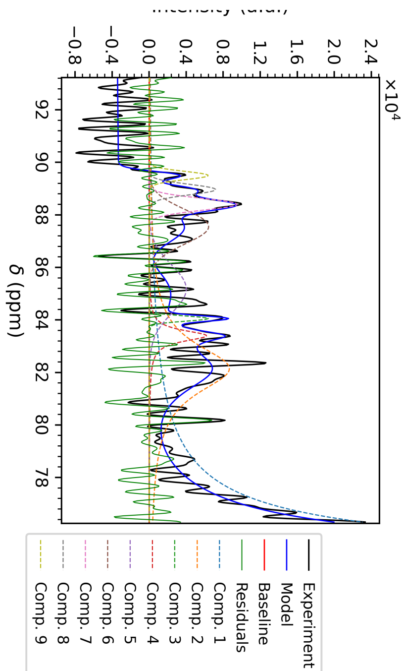
Figure 3.24: Fit della zona dei C 4 dell'involucro di Vespa vulgaris (800 MHz)
