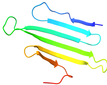
Figure 3.2: Struttura della proteina PdomMRNAr1.2-08705.1 eliminando la porzione ad alfa elica
