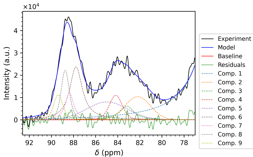
Figure 3.18: Fit della zona dei C 4 del campione più nuovo di Polistes dominula (800 MHz)
