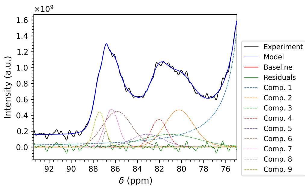
Figure 3.19: Fit della zona dei C 4 del campione più vecchio di Polistes gallicus (700MHz)
