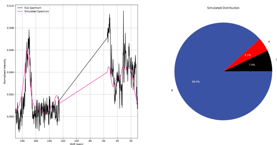
Figure 3.25: Predizione del segnale proteico sullo spettro di Polistes dominula
