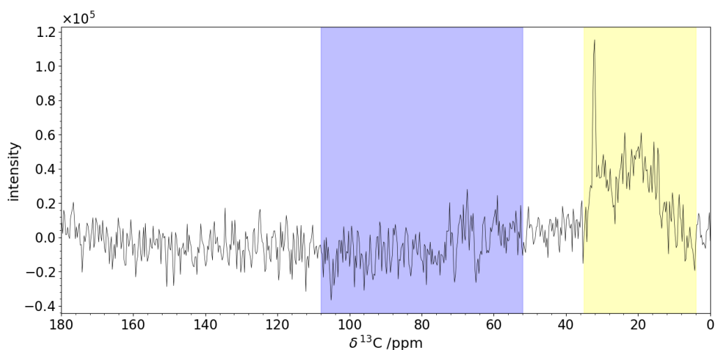
Figure 2.12: Prima traccia del segnale del protone Polistes dominula
