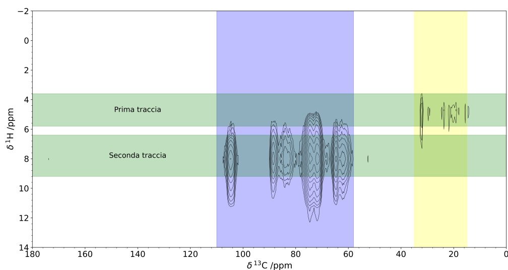
Figure 2.11: Spettro bidimensionale Polistes dominula
