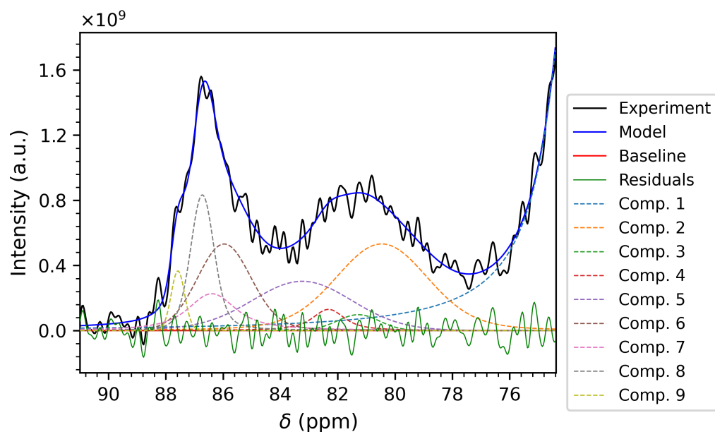
Figure 3.16: Fit della zona dei C 4 del campione più vecchio di Polistes dominula (700 MHz)
