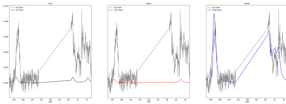
Figure 3.26: Contribuzione del segnale da parte delle differenti strutture secondarie
