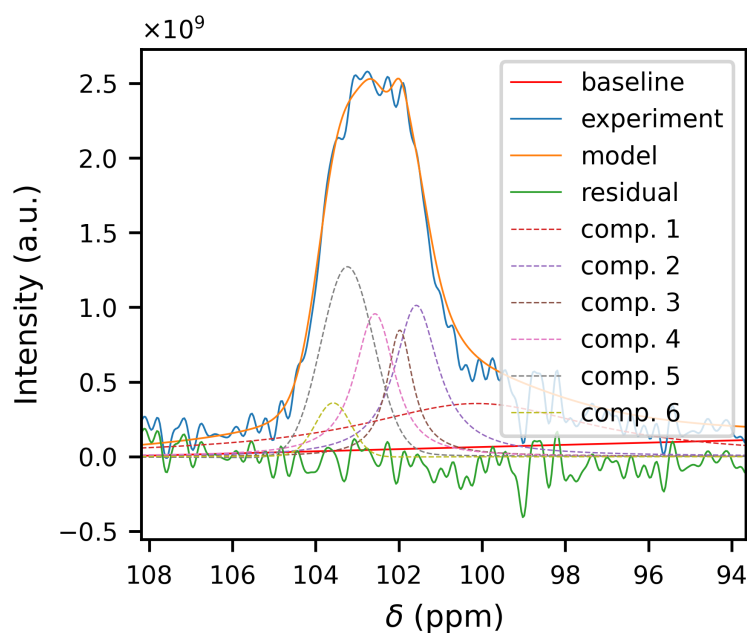
Figure 3.7: Fit della zona dei C1 per il campione più vecchio di Polistes dominula (700 MHz)
