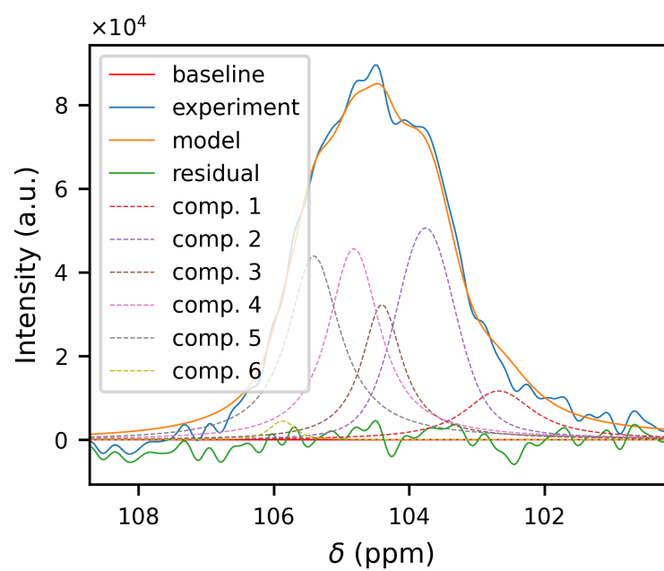
Figure 3.9: Fit della zona dei C1 per il campione più nuovo di Polistes dominula (800 MHz)
