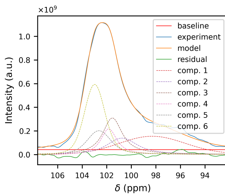
Figure 3.11: Fit della zona dei C1 per il campione più nuovo di Polistes gallicus (700 MHz)
