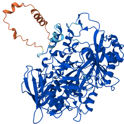
Figure 1.4: Struttura della proteina PdomMRNAr1.2-10508.1 predetta con Alphafold
