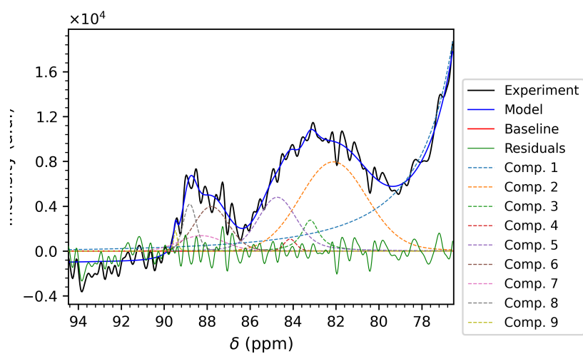
Figure 3.23: Fit della zona dei C 4 delle celle di Vespula vulgaris (800 MHz)
