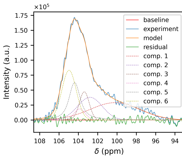
Figure 3.12: Fit della zona dei C1 per le celle di Vespa crabro (800 MHz)
