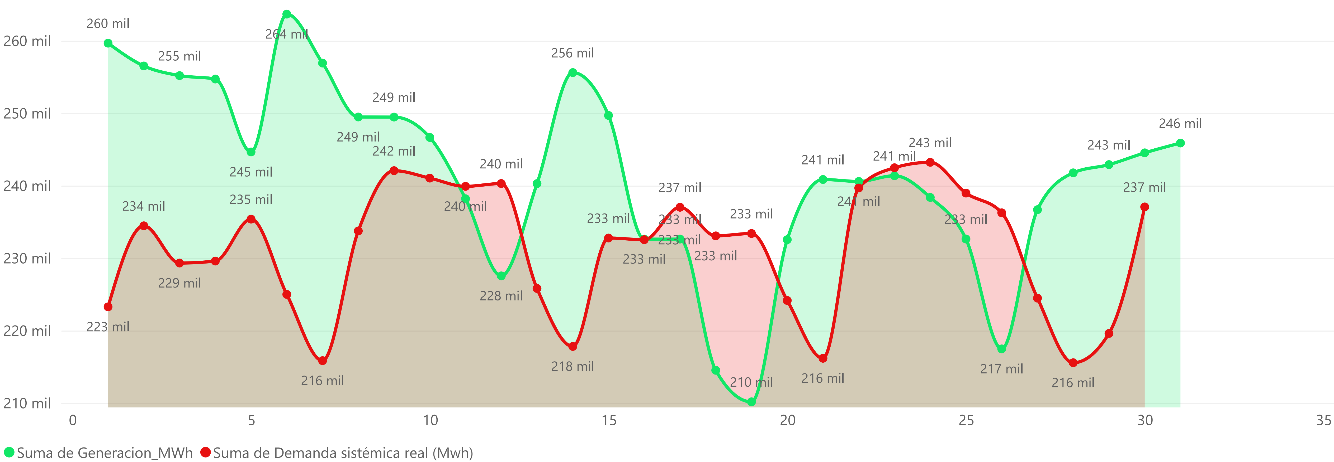
Suma de Generacion_MWh y Suma de Demanda sistémica real (Mwh) por Día
