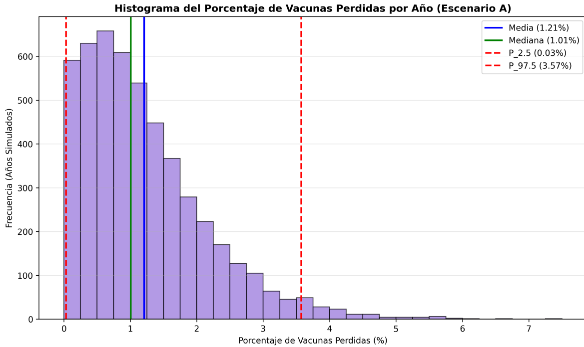
Figura 4.21: Histograma del porcentaje de vacunas perdidas anualmente (Escenario A). La distribución presenta una fuerte asimetría positiva (una cola larga estirada hacia la derecha). Esto indica que, aunque la concentración principal de los datos sugiere pérdidas bajas (mediana del 1.01 %), existen años atípicamente catastróficos que arrastran el promedio general hacia arriba (1.21 %). Las líneas rojas punteadas delimitan el intervalo empírico del 95 %, mostrando la alta dispersión hacia escenarios extremos.
