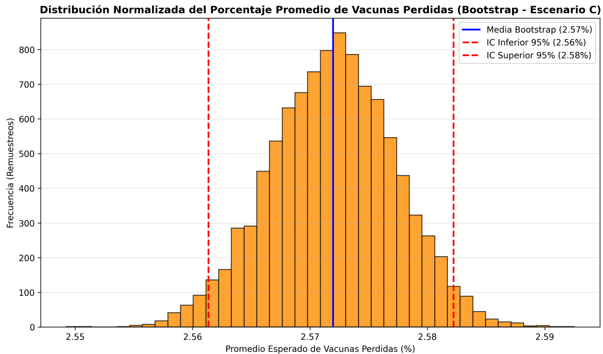
Figura 4.29: Distribución normalizada del porcentaje de pérdida (Escenario C). La campana se establece en el nivel más crítico del análisis, confirmando con absoluta precisión geométrica que la pérdida poblacional esperada es del 2.57 %, acotada estrictamente entre el 2.56 % y el 2.58 %.
