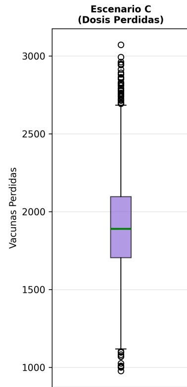
Figura 4.26: Diagrama de caja de dosis perdidas (Escenario C). La caja se posiciona en un nivel de destrucción extremo. A diferencia de los escenarios anteriores, el aumento masivo de la varianza provoca que aparezcan valores atípicos tanto en la cola superior (superando las 3,000 dosis) como en la inferior (cayendo a 1,000 dosis), confirmando la forma de campana observada en su histograma.
