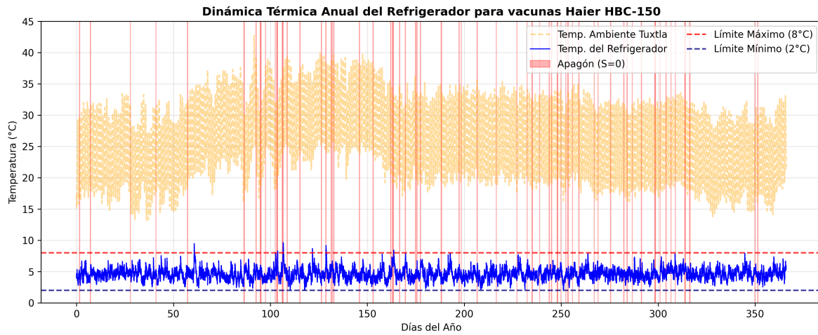
Figura 5.1: Dinámica térmica anual simulada para el refrigerador Haier HBC-150. Las zonas sombreadas en rojo indican la ocurrencia de los 68 apagones a lo largo del año, la trayectoria de color azul indica la temperatura interna del refrigerador (la solución numerica de la EDE), y la trayectoria de color amarillo inidica la temperatura ambiente en Tuxtla Gutiérrez, Chiapas.
