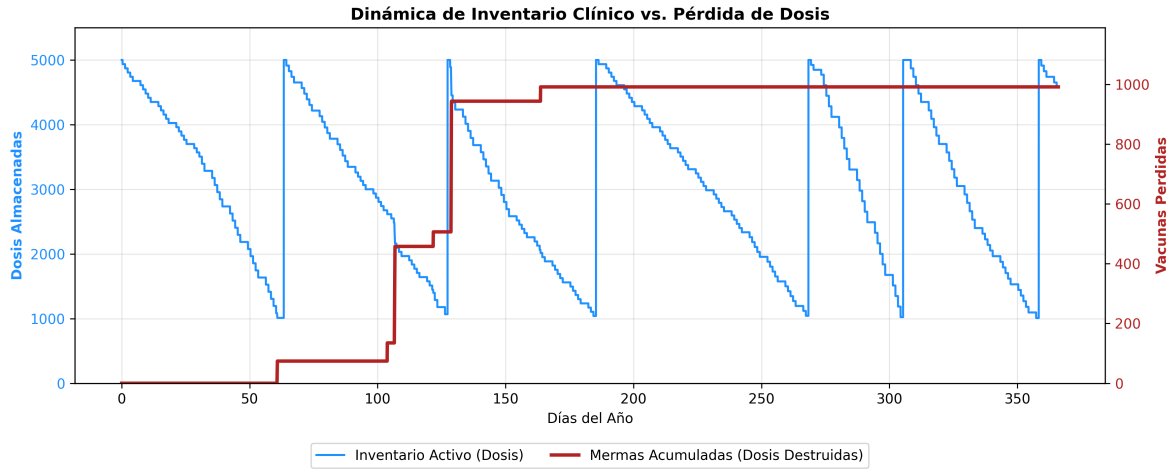
Figura 5.3: Simulación del inventario de vacunas a lo largo del año (dientes de sierra) de la central de almacenamiento de vacunas (eje izquierdo) y el crecimiento acumulado de las dosis destruidas por fallas térmicas (eje derecho).
