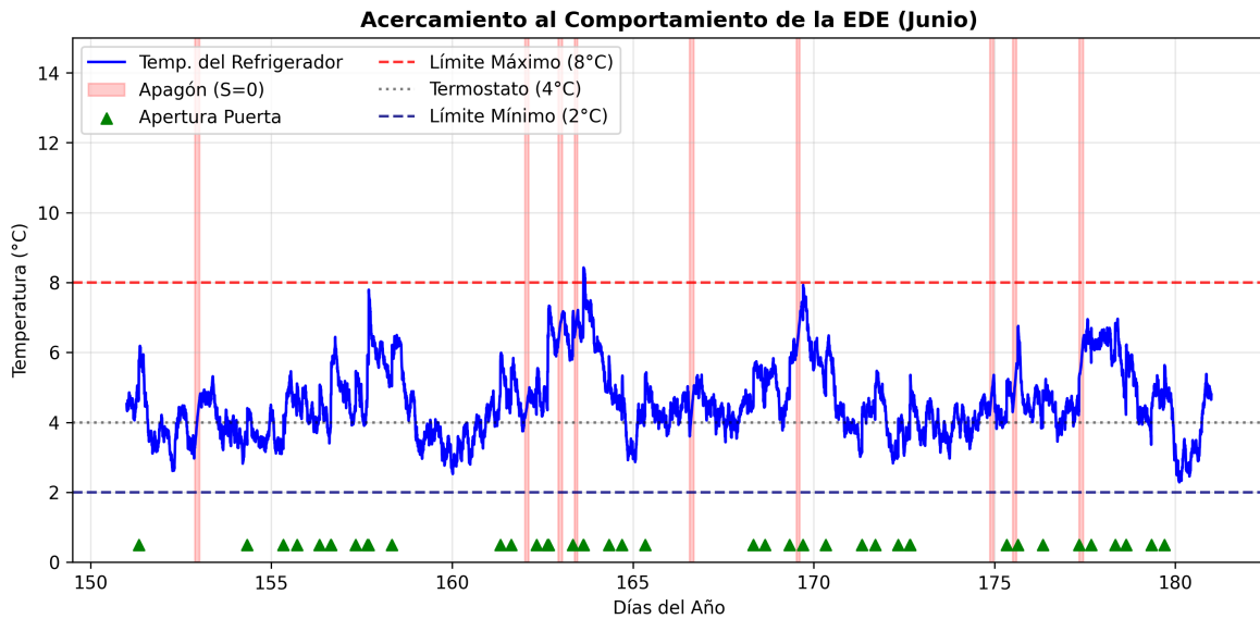
Figura 5.2: Acercamiento del comportamiento de la EDE durante el mes de junio. Se omitió el clima exterior para observar la estabilidad del termostato ( 4^{\circ}\text{C} ), los impactos de las aperturas (triángulos verdes inferiores) y la pérdida de frío en los apagones.
