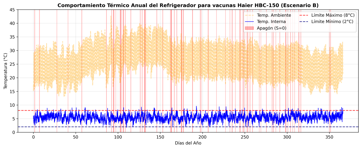
Figura 4.4: Comportamiento térmico anual (Escenario B). La interacción humana controlada engrosa la trayectoria azul, incrementando los picos térmicos debido a las aperturas matutinas y vespertinas.
