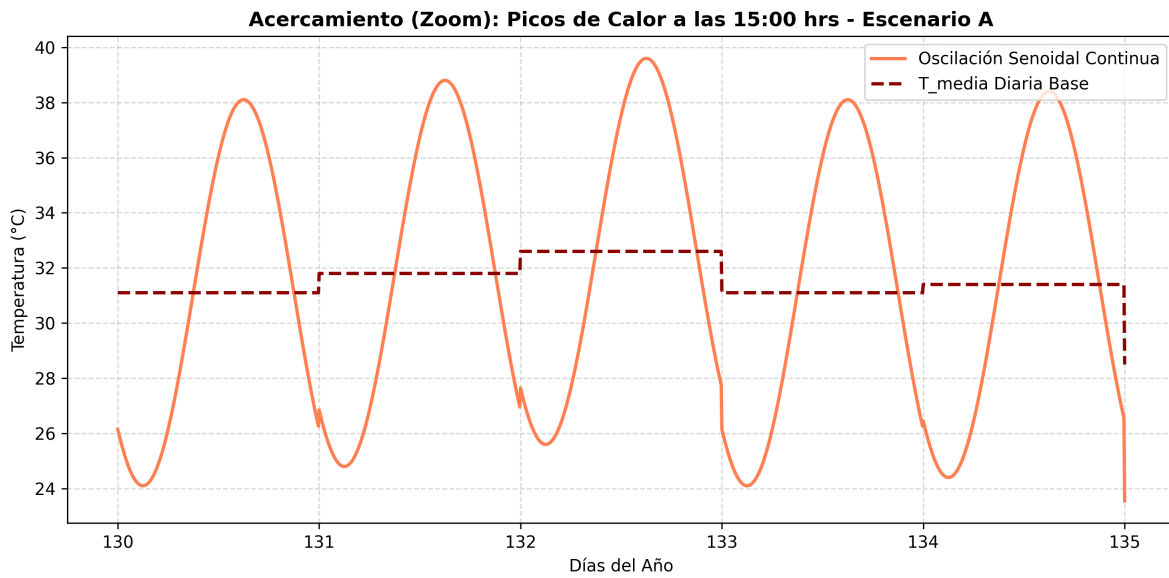
Figura 4.2: Acercamiento a un periodo de 5 días de simulación climática (Mayo), donde se observa el ciclo senoidal y los picos térmicos a las 15:00 horas.
