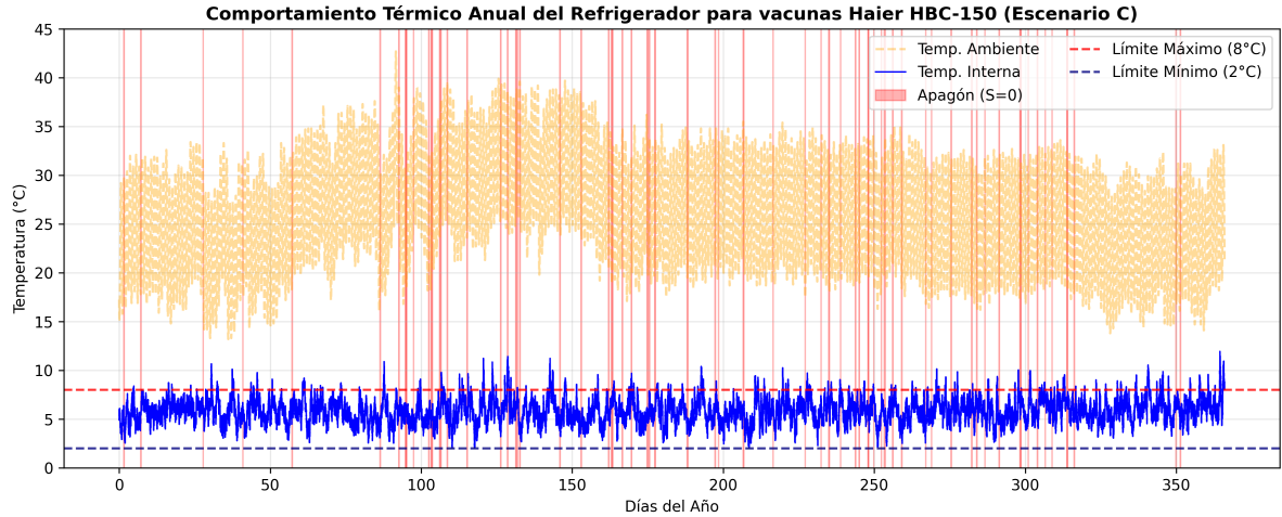
Figura 4.5: Comportamiento térmico anual (Escenario C). La saturación logística colapsa el control termodinámico; la trayectoria azul se muestra muy oscilatoria, rompiendo continuamente la barrera de los 8°C.
