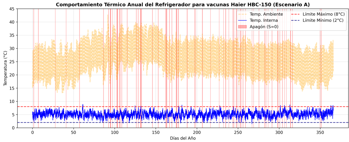
Figura 4.3: Comportamiento térmico anual (Escenario A). Las zonas sombreadas en rojo indican la ocurrencia de los 68 apagones. La trayectoria azul representa la temperatura interna del equipo (la solución numérica de la EDE) la cual se mantiene estable y rara vez rompe la cadena de frío, viéndose afectada únicamente por fallas eléctricas prolongadas, y la trayectoria de color amarillo indica la temperatura ambiente en Tuxtla Gutiérrez, Chiapas.
