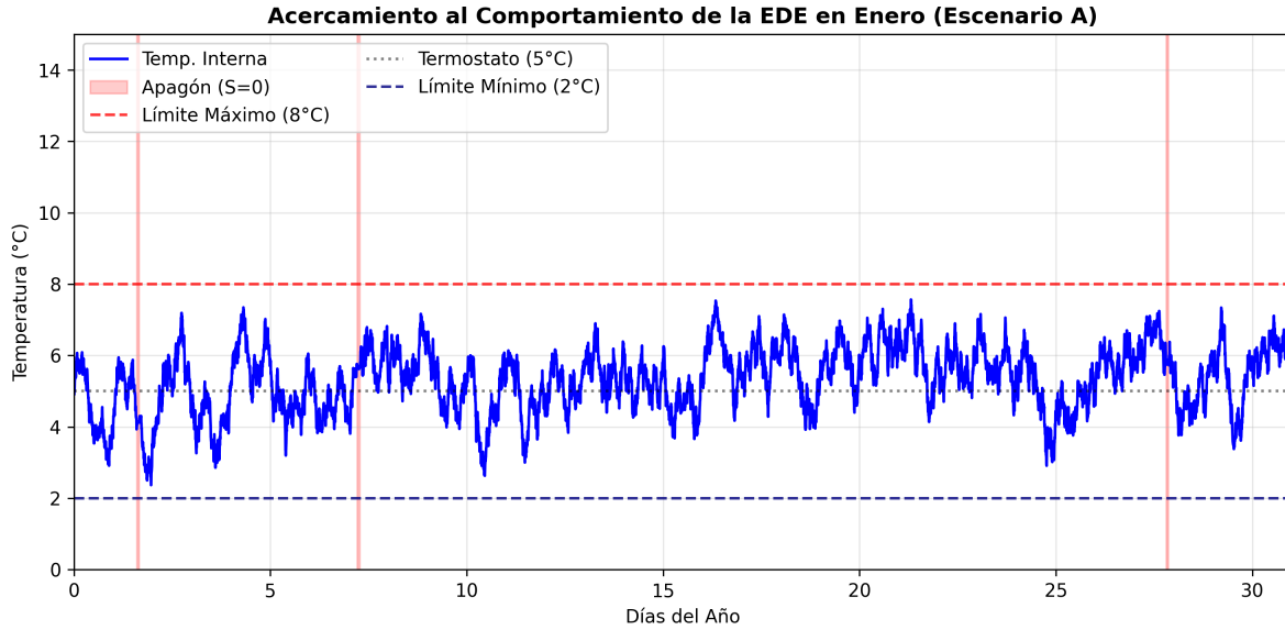
Figura 4.6: Acercamiento del comportamiento de la EDE durante el mes de enero (Escenario A). Se omitió el clima exterior para observar la estabilidad del termostato ( 5^{\circ}\text{C} ), sin la presencia de personal clínico, las únicas perturbaciones observables son curvas suaves de calentamiento pasivo durante los cortes de energía.
