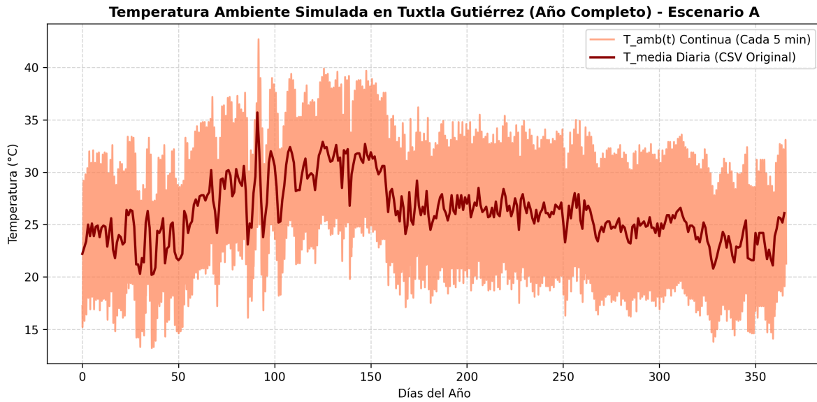
Figura 4.1: Temperatura ambiente continua simulada para Tuxtla Gutiérrez a lo largo de un año, comparada con los promedios diarios de la base meteorológica.
