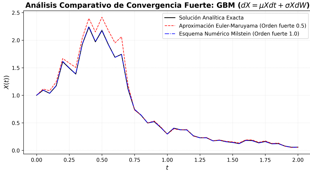
Figura 2.4: Análisis de convergencia fuerte de esquemas numéricos estocásticos para una trayectoria de Movimiento Browniano Geométrico (GBM) definida por dX = 0.05Xdt + 0.4X dW con X_0 = 1 . El eje horizontal representa el tiempo discreto y el eje vertical el estado del proceso X(t) . La línea negra continua muestra la solución analítica exacta. La línea roja discontinua ilustra la aproximación de Euler-Maruyama (Orden fuerte 0.5), evidenciando desviaciones significativas y oscilaciones erráticas respecto a la trayectoria real. La línea azul discontinua-punto representa el esquema de Milstein (Orden fuerte 1.0), el cual sigue con alta precisión la dinámica exacta, demostrando su estabilidad superior ante ruidos multiplicativos y mallados temporales gruesos. La fuente de los datos corresponde a una simulación de elaboración propia generada en Python.
