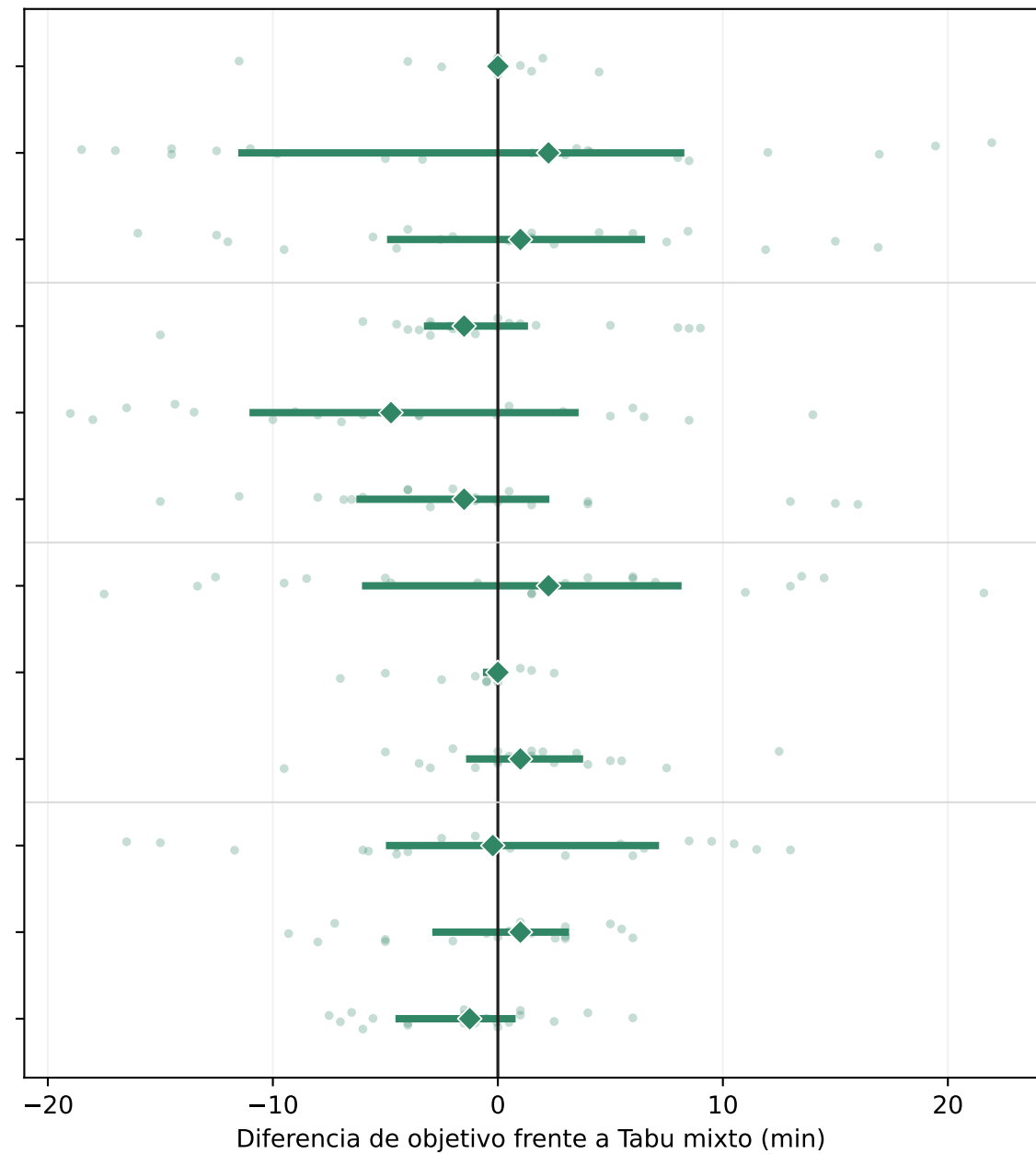
Tabu + UCB1
