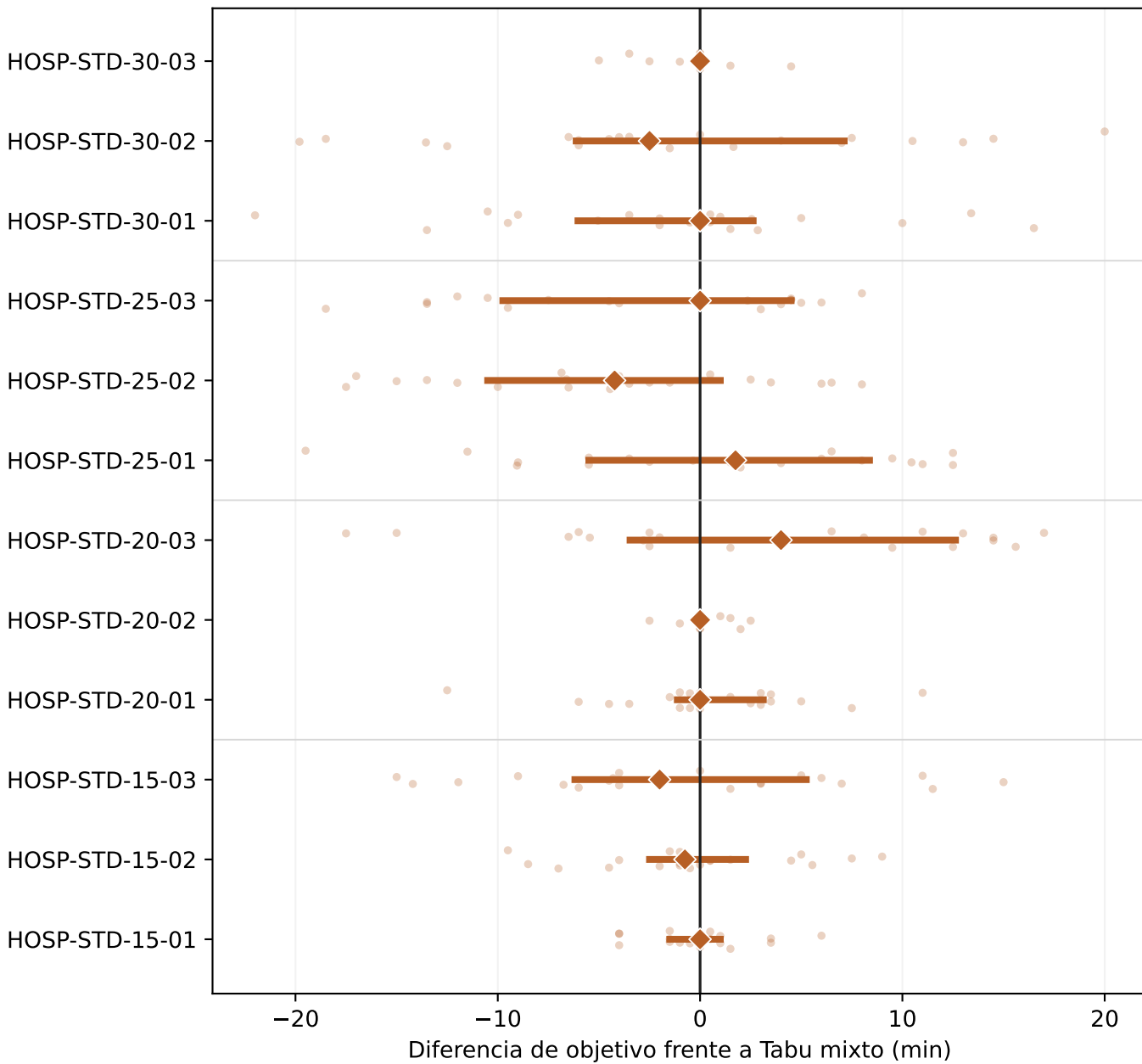
Tabu + D-MAB
