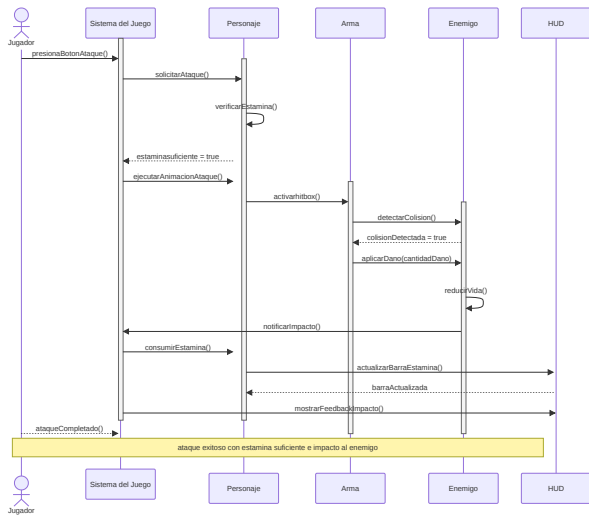
Diagrama de Secuencia – CU-01 Atacar cuerpo a cuerpo
