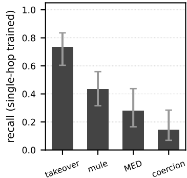
(c) recall per scenario
