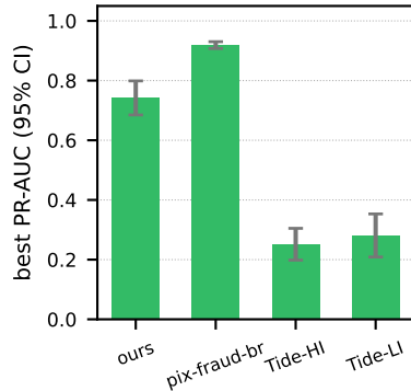
(d) PR-AUC per source
