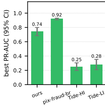
(d) PR-AUC per source
