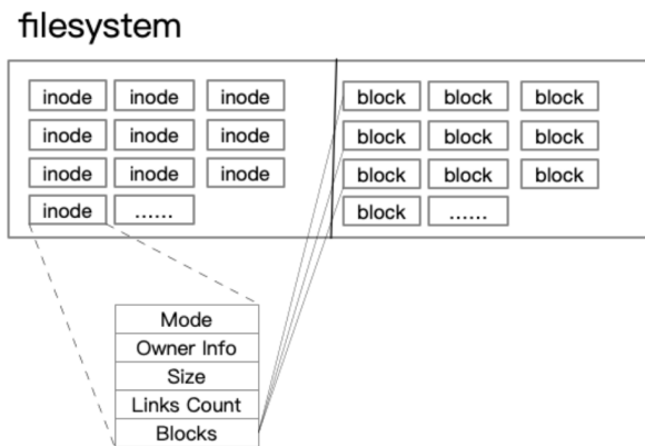
Figura 12.1: Il Linux iNode
