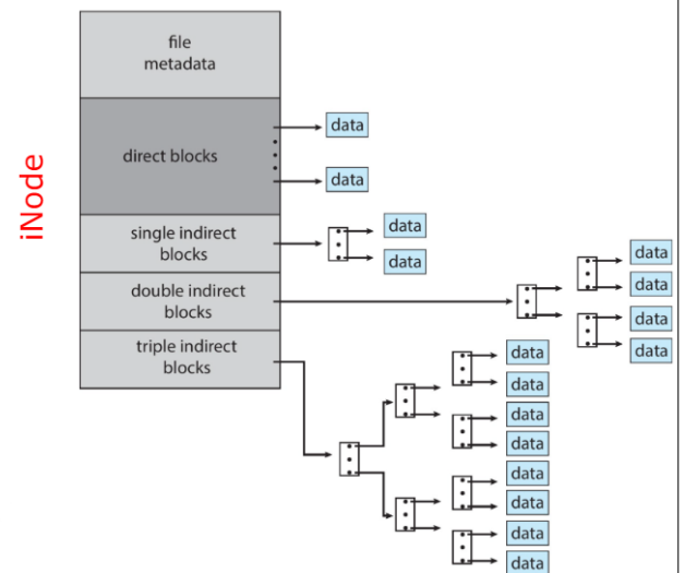
Figura 12.2: UNIX UFS - 4 KB per blocco, indirizzi a 32 bit
