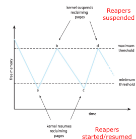
Figura 14.7: Esempio di recupero delle pagine
