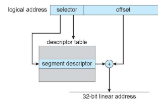
Figura 15.6: Conversione degli indirizzi di memoria
