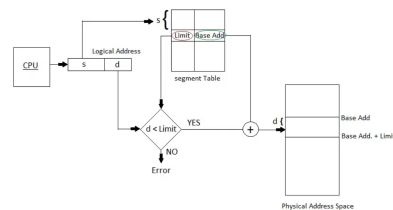
Figura 15.5: Segmentazione: da logico a fisico
