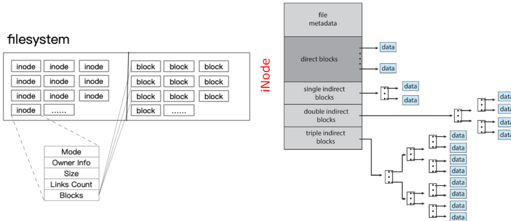
Figura 19.1: Il Linux iNode
