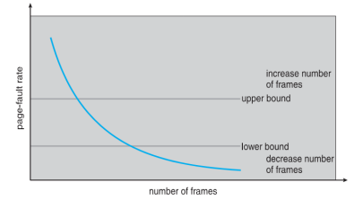
Figura 14.8: PFF
