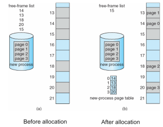
Figura 14.3: Frame liberi
