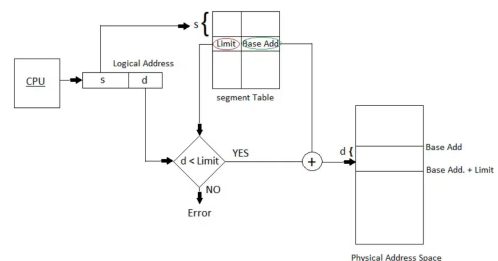
Figura 14.5: Segmentazione: da logico a fisico
