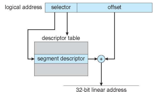
Figura 14.6: Conversione degli indirizzi di memoria
