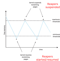
Figura 13.8: Esempio di recupero delle pagine
