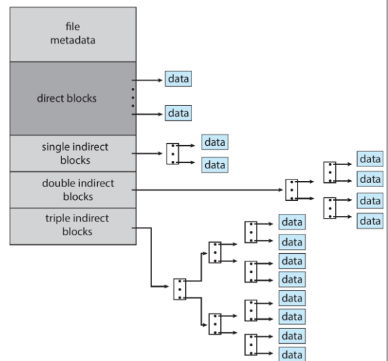
Figura 18.2: UNIX UFS - 4 KB per blocco, indirizzi a 32 bit
