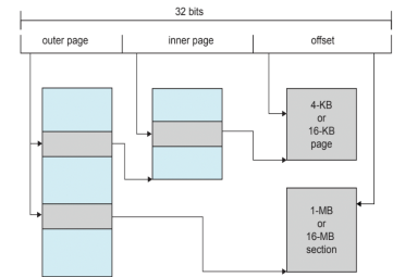
Figura 14.7: Architettura ARM
