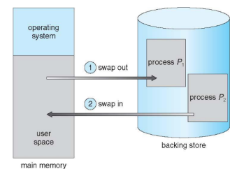
Figura 14.1: Processo di swapping
