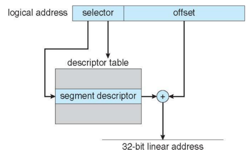
Figura 11.6: Conversione degli indirizzi di memoria
