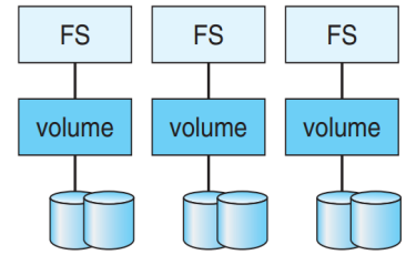
Figura 12.5: Volumi e file system tradizionali
