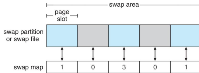
Figura 12.2: Strutture dati per lo swapping nei sistemi Linux
