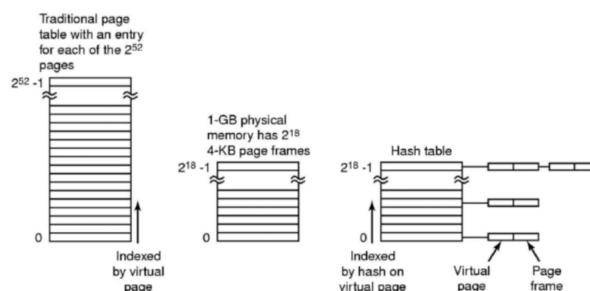
Figura 11.4: Comparativa tra tabella delle pagine tradizionale e tabella delle pagine invertita
