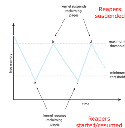
Figura 10.8: Esempio di recupero delle pagine
