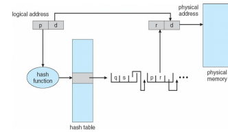
Figura 11.3: Tabella delle pagine con hashing
