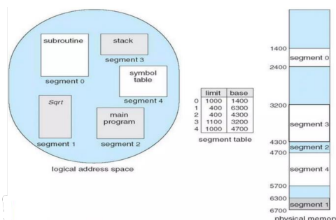
Figura 11.5: Segmentazione: da logico a fisico
