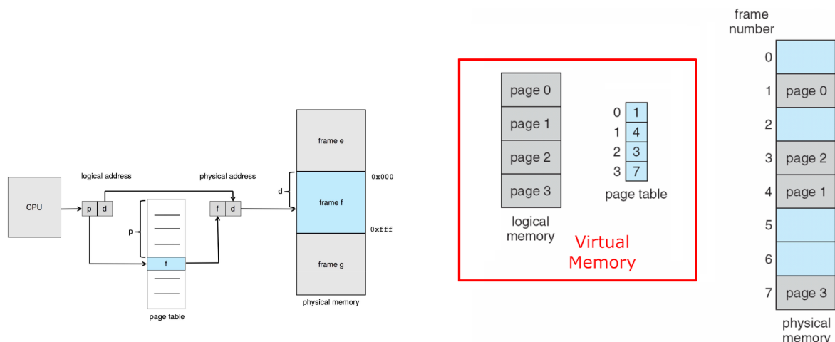
Figura 10.3: Modello di paginazione della memoria logica e fisica
