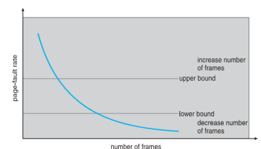
Figura 8.9: PFF
