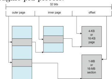
Figura 9.7: Architettura ARM
