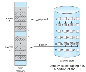
Figura 10.2: Swapping con paginazione
