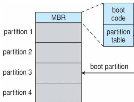
Figura 11.1: Avvio dallo storage secondario in Windows
