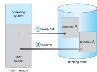
Figura 10.1: Processo di swapping
