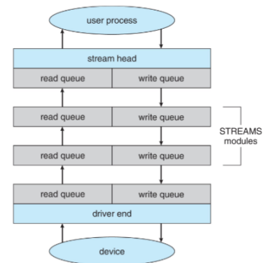
Figura 13.2: La struttura degli STREAMS
