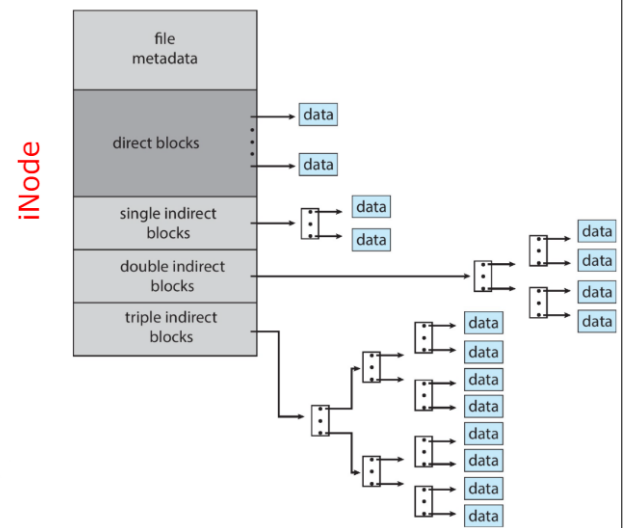
Figura 14.2: UNIX UFS - 4 KB per blocco, indirizzi a 32 bit
