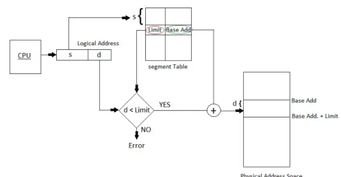
Figura 10.5: Segmentazione: da logico a fisico
