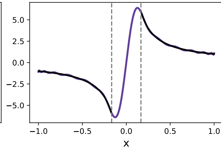
d=25, \varepsilon \approx 0.088
