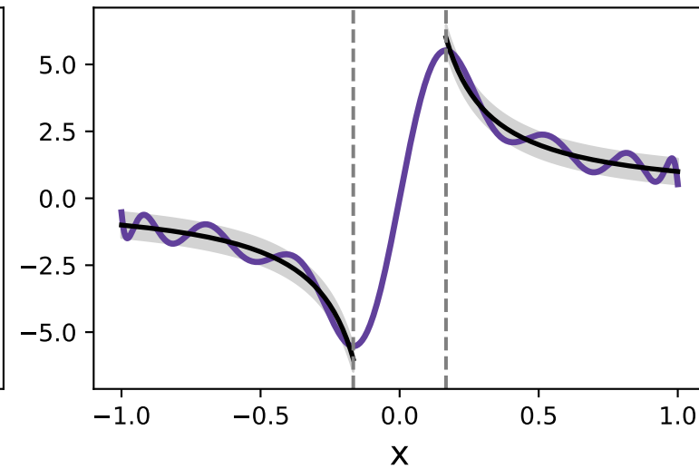
d=15, \varepsilon \approx 0.47
