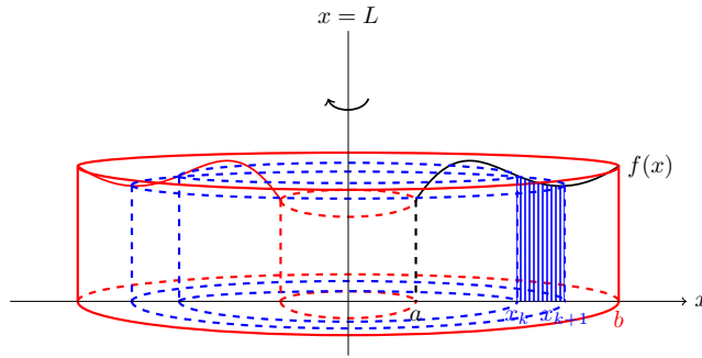
Figure 4: Representación esquemática del sólido de revolución S (en color rojo) obtenido al rotar el área encerrada por la curva f(x) , y las rectas x = a e x = b , entorno a la recta x = L .
