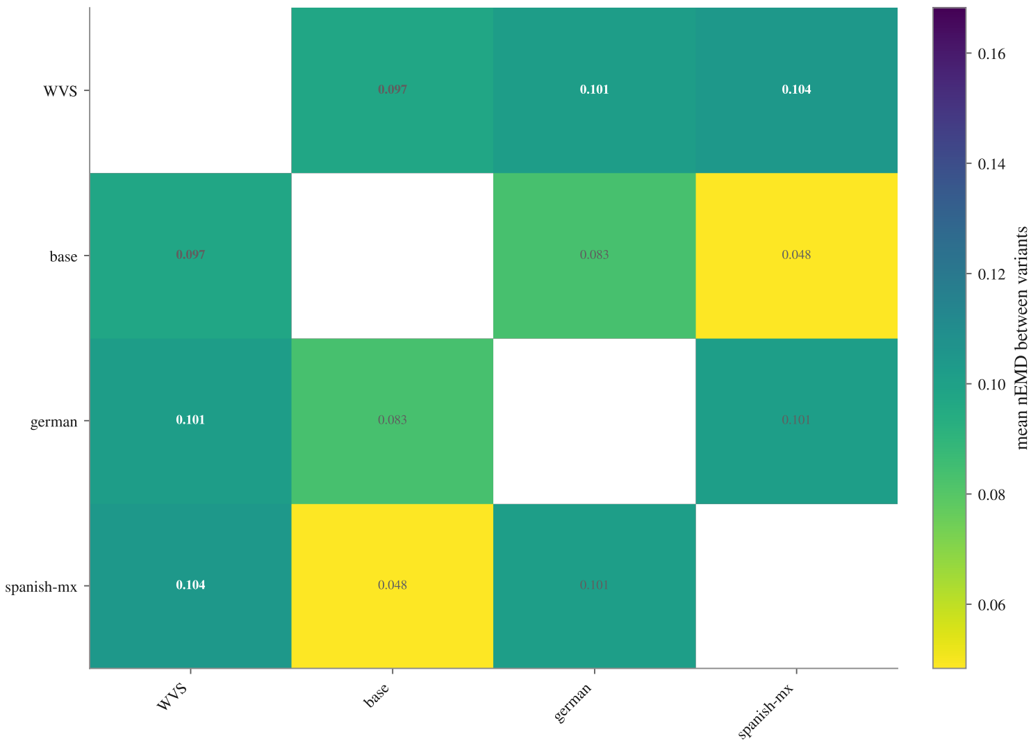
Llama-3.2-3B
