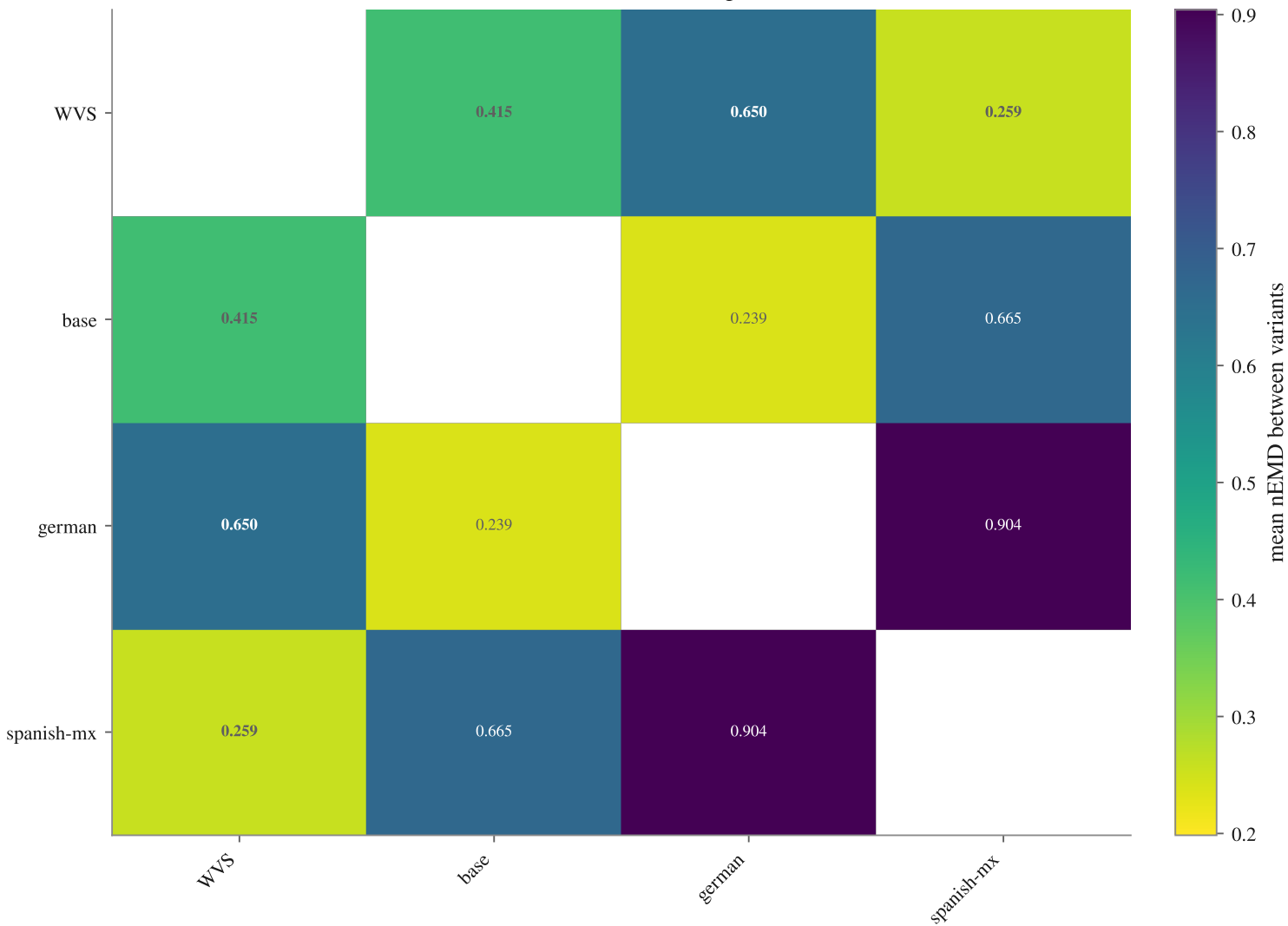
Qwen3-VL-2B-Thinking
