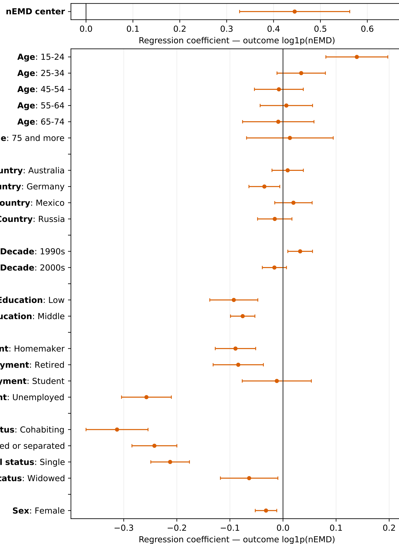
NTP (adj. R^2 = 0.508 )
