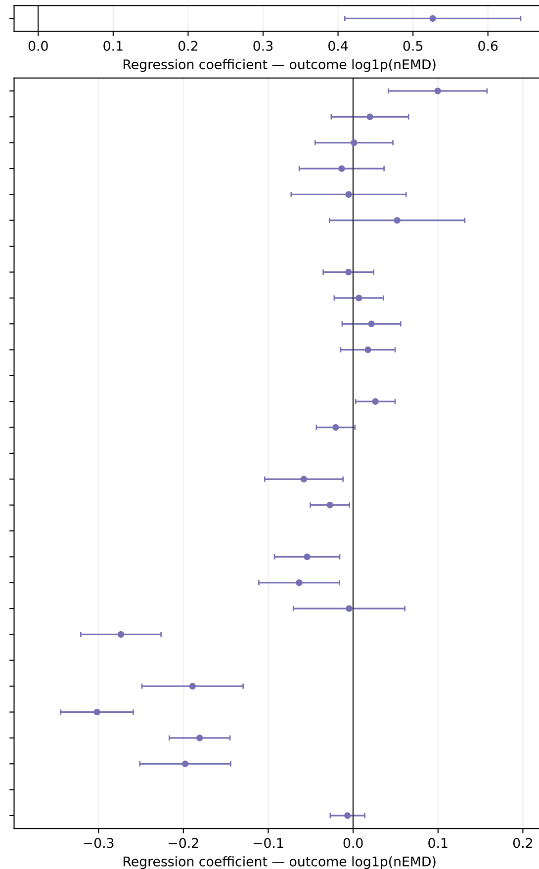
FA (adj. R^2 = 0.540 )
