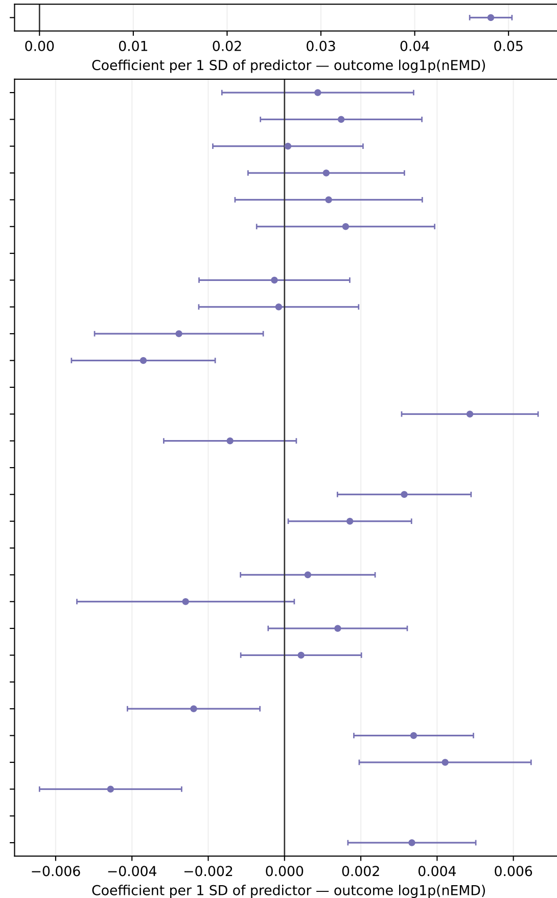
FA (adj. R^2 = 0.862 )
