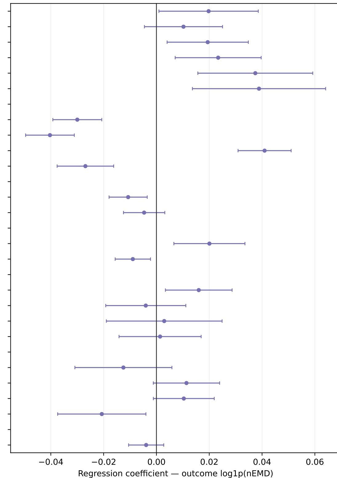
FA (adj. R^2 = 0.450 )
