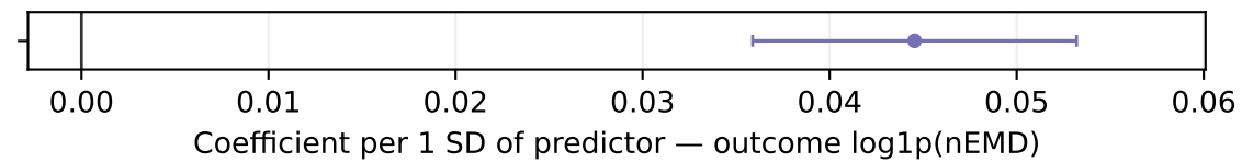
FA (adj. R^2 = 0.619 )
