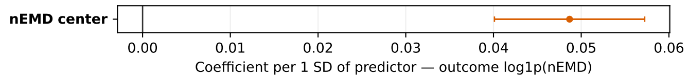
NTP (adj. R^2 = 0.641 )
