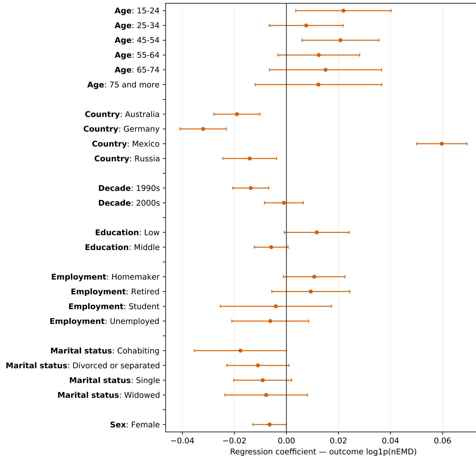
NTP (adj. R^2 = 0.496 )
