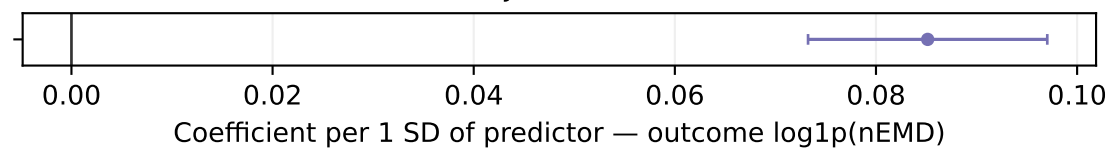
FA (adj. R^2 = 0.740 )
