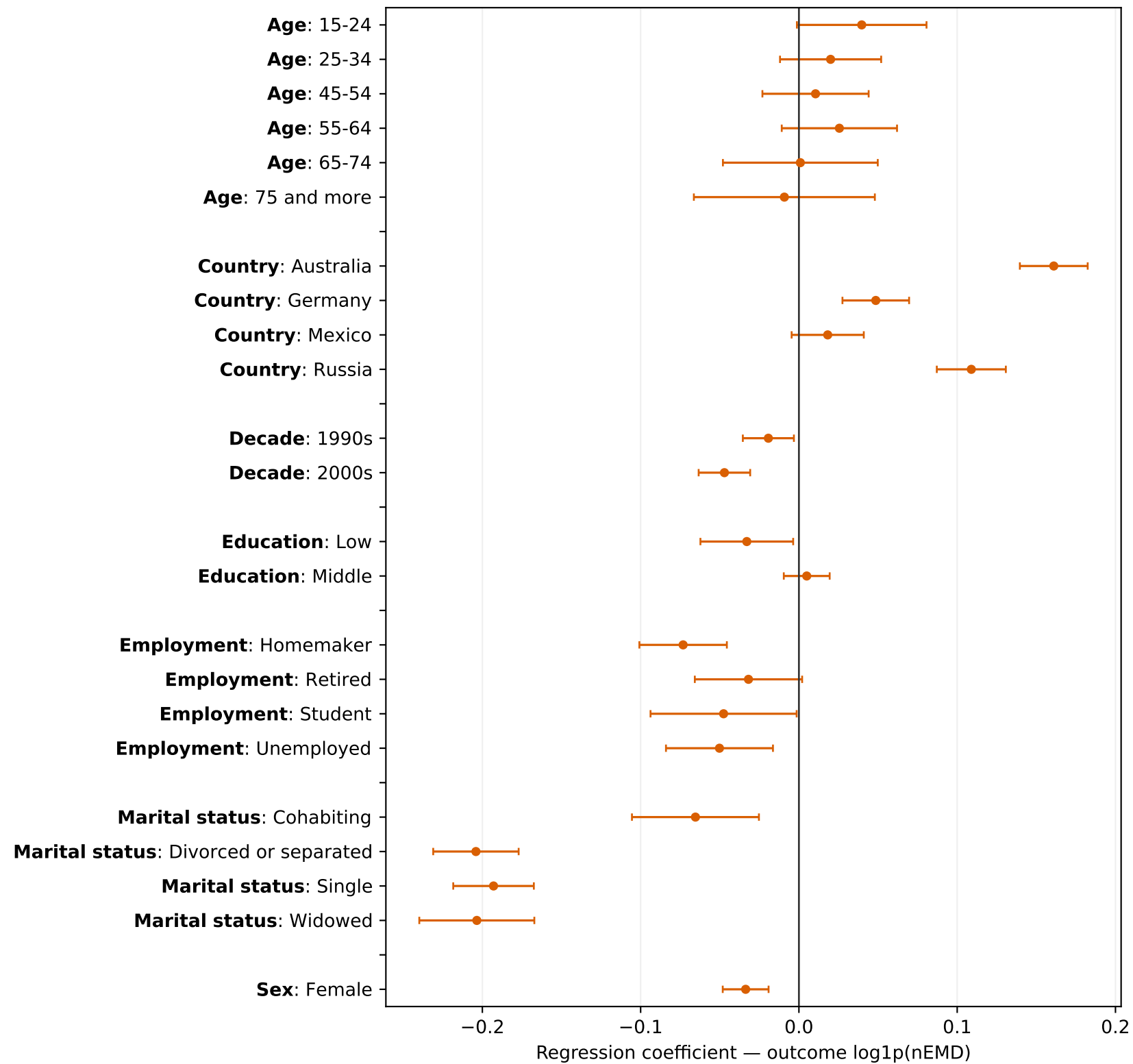
NTP (adj. R^2 = 0.658 )
