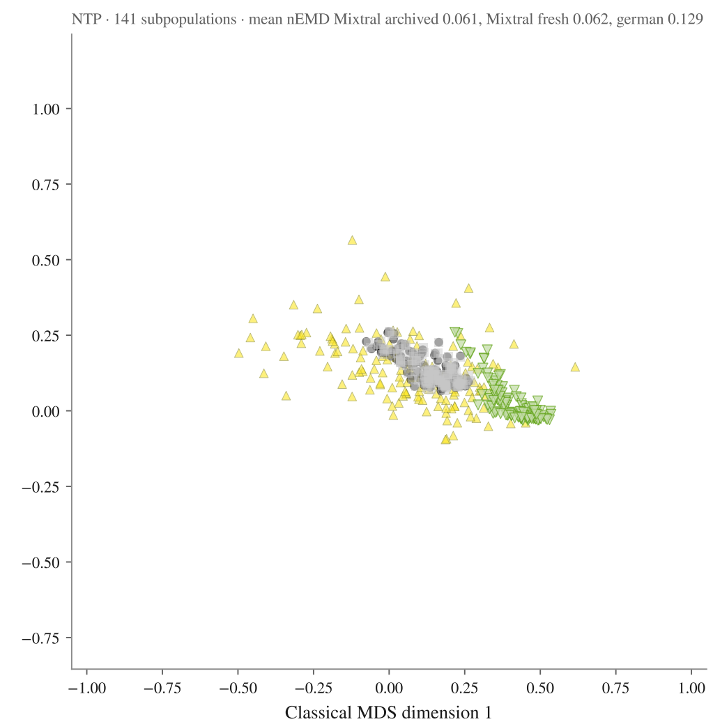
Qwen3-VL-8B-Thinking
