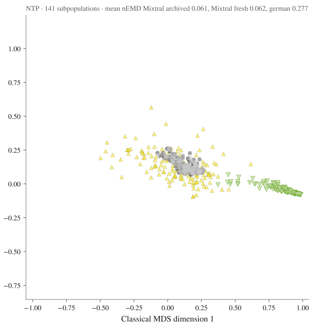
Gemma-4-E4B-it
