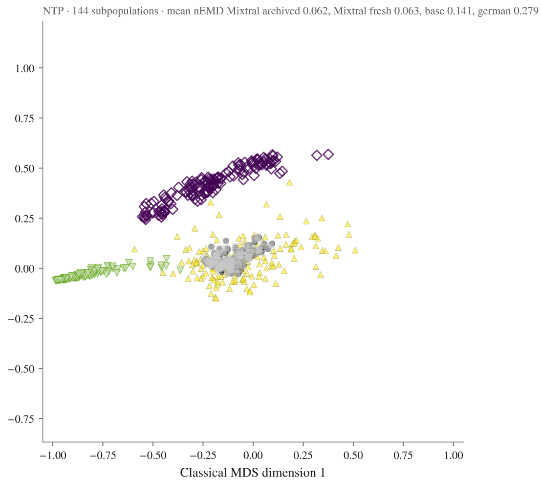
Llama-3.2-3B
