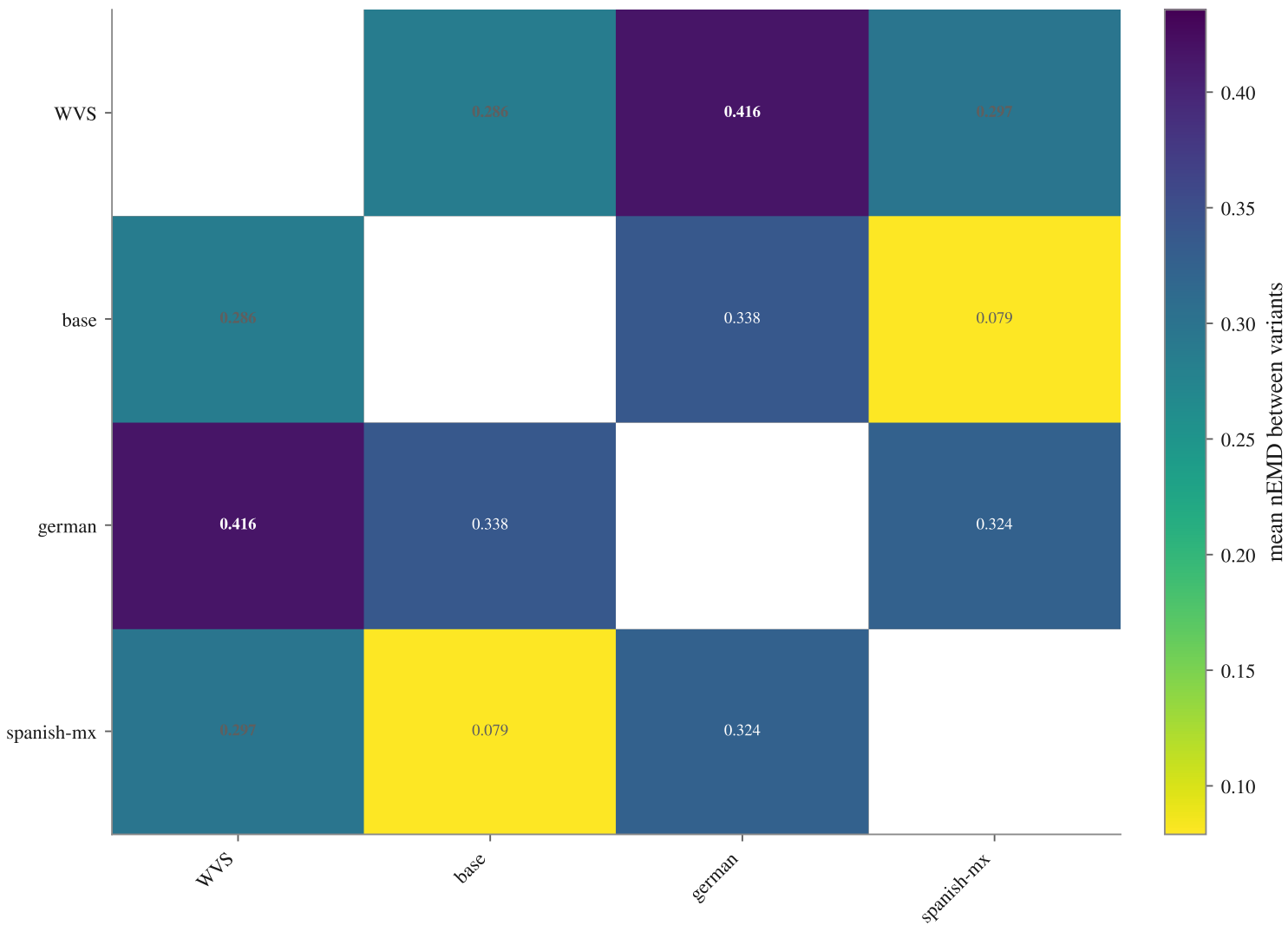
Gemma-4-31B-it
