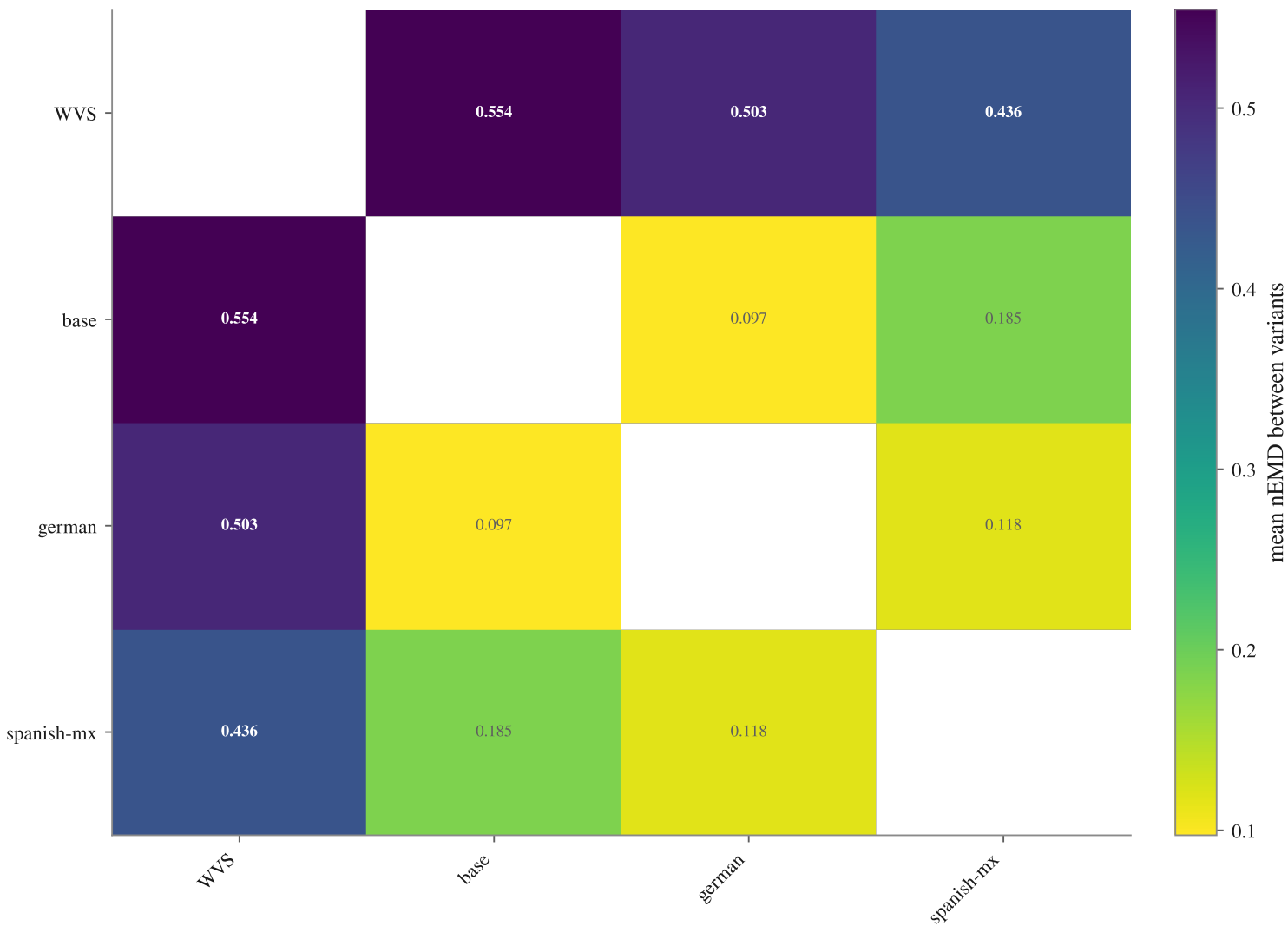
Gemma-4-E4B-it
