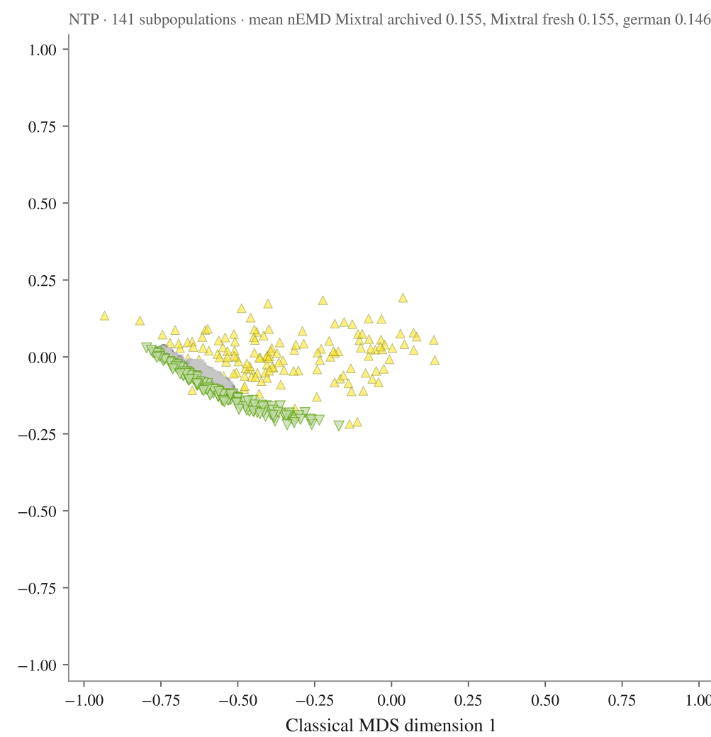
Qwen3-VL-8B-Thinking
