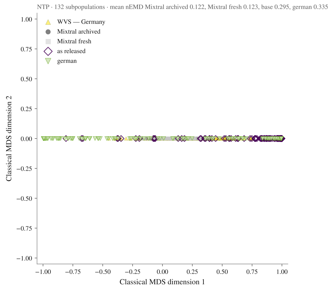
Gemma-4-31B-it
