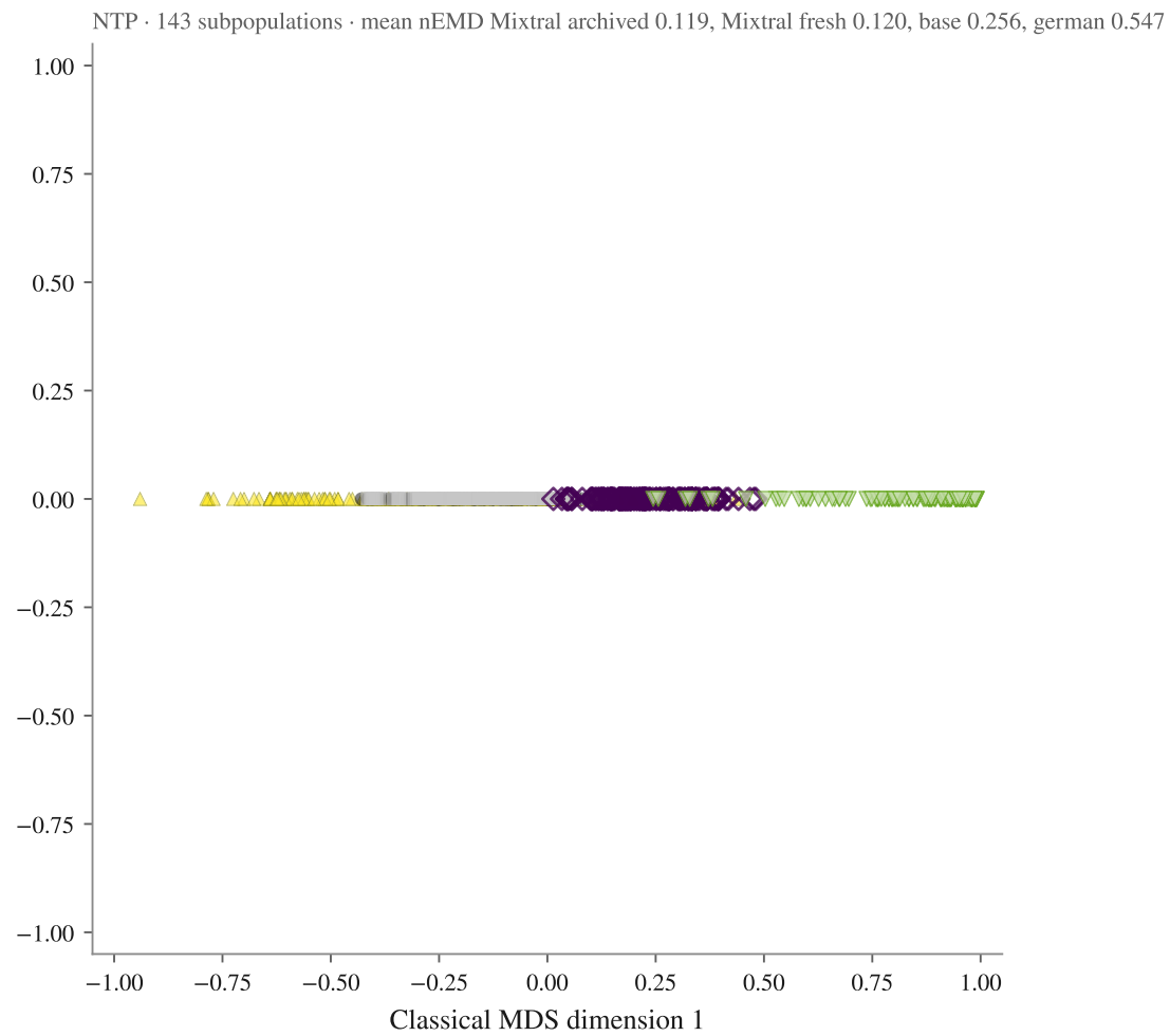
Llama-3.2-3B
