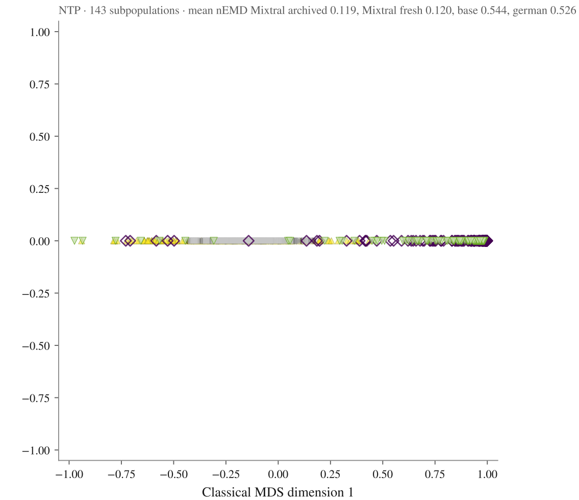
Gemma-4-E4B-it
