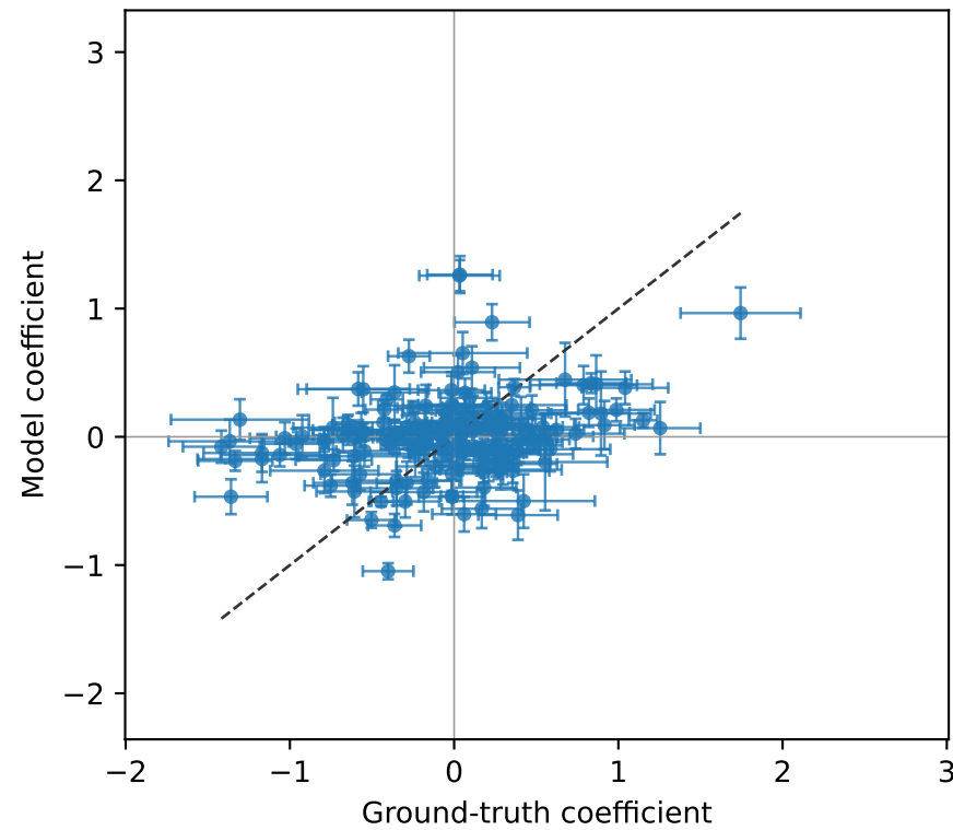
FA-GPT-3
