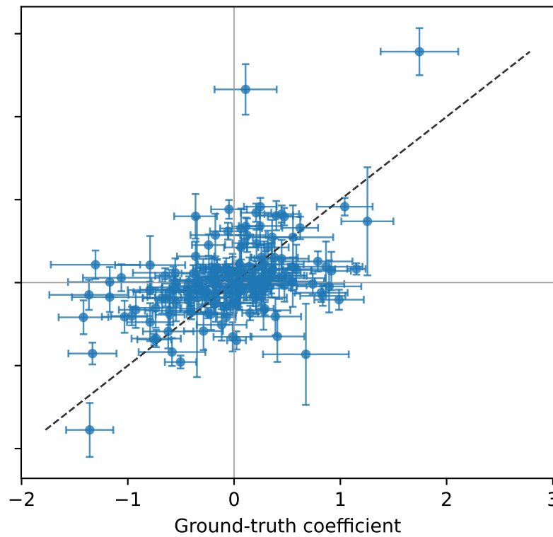
FA-Llama-3-70B
