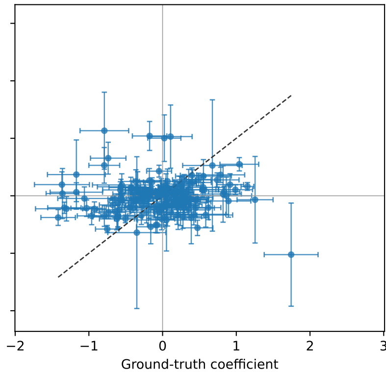
FA-Mixtral-8x7B
