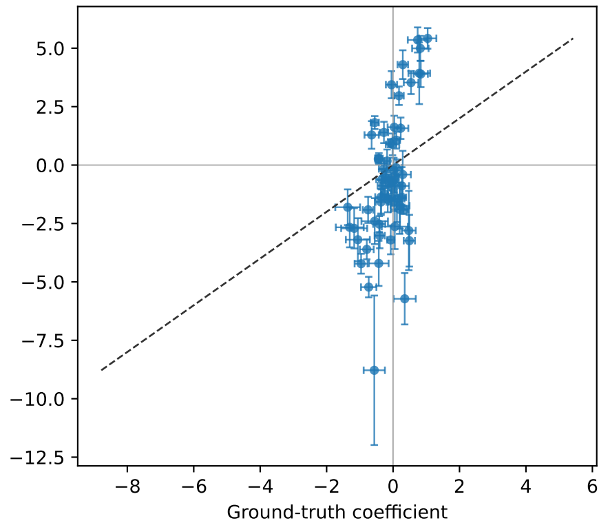
NTP-GPT-4T
