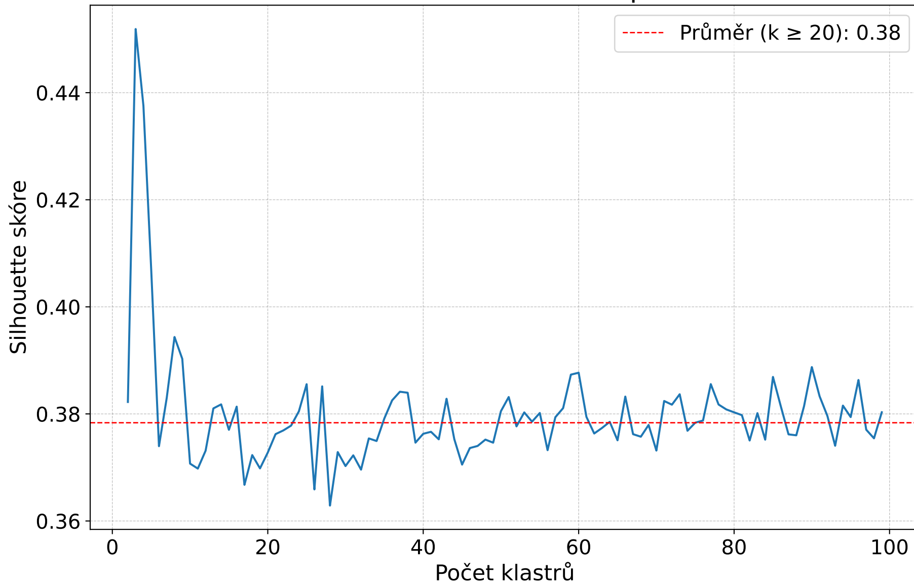
Silhouette skóre v závislosti na počtu klastrů
