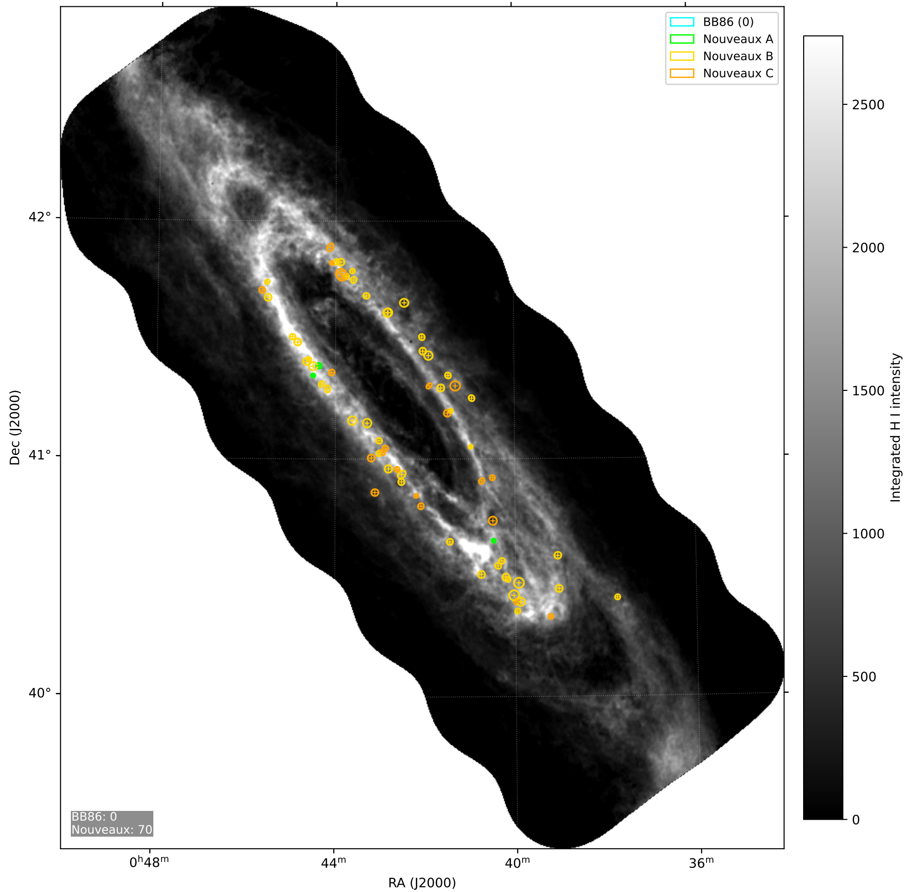
M31 — cavités BB86 et nouveaux candidats H I
