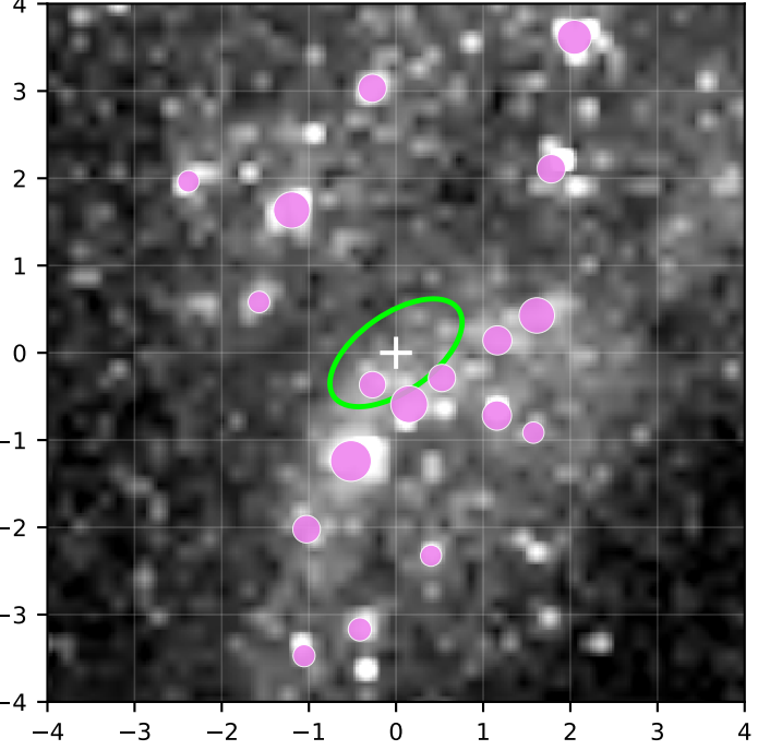
GALEX FUV
