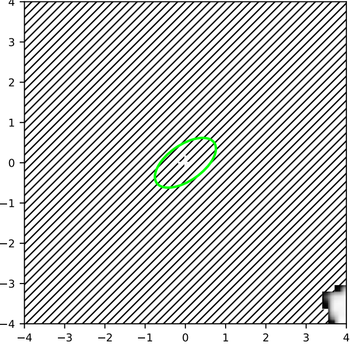
PHAST F814W
