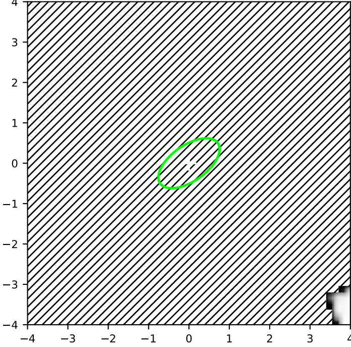
PHAST F475W
