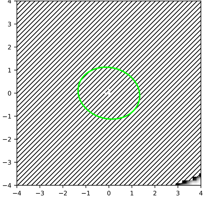
PHAST F814W
