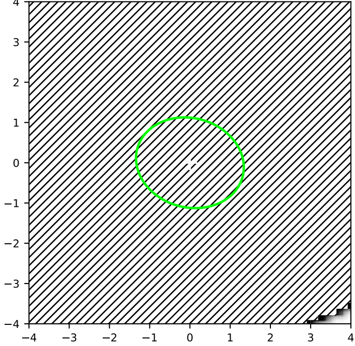
PHAST F475W
