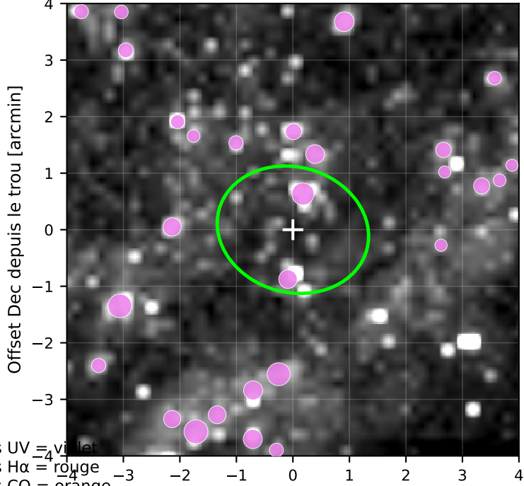
GALEX NUV
