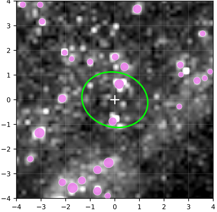
GALEX FUV
