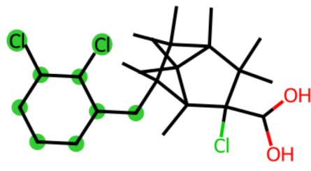
Pred: di_chloro_ortho
