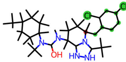
Pred: di_chloro_meta
