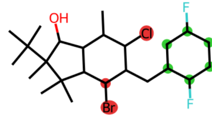
Pred: di_fluoro_para
