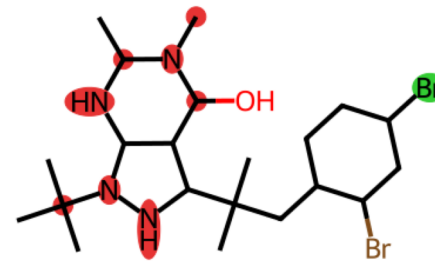
Pred: di_bromo_meta
