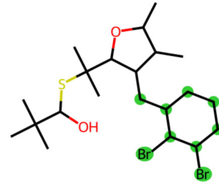
Pred: di_bromo_ortho
