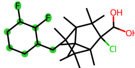
Pred: di_fluoro_ortho
