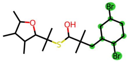
Pred: di_bromo_para
