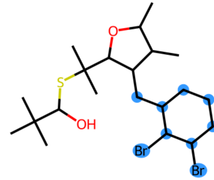
di_bromo_ortho
