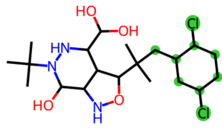
Pred: di_chloro_para
